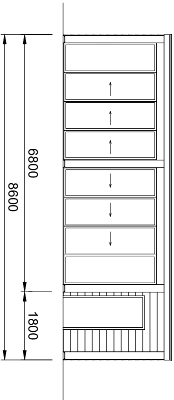
vooraanzicht
