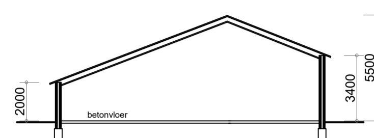
- Doorsnede B - B gebouw 3 -
