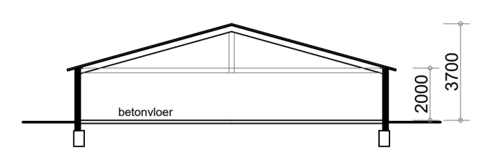
- Doorsnede C - C gebouw 4 -
