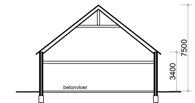
- Doorsnede A - A gebouw 2 -
