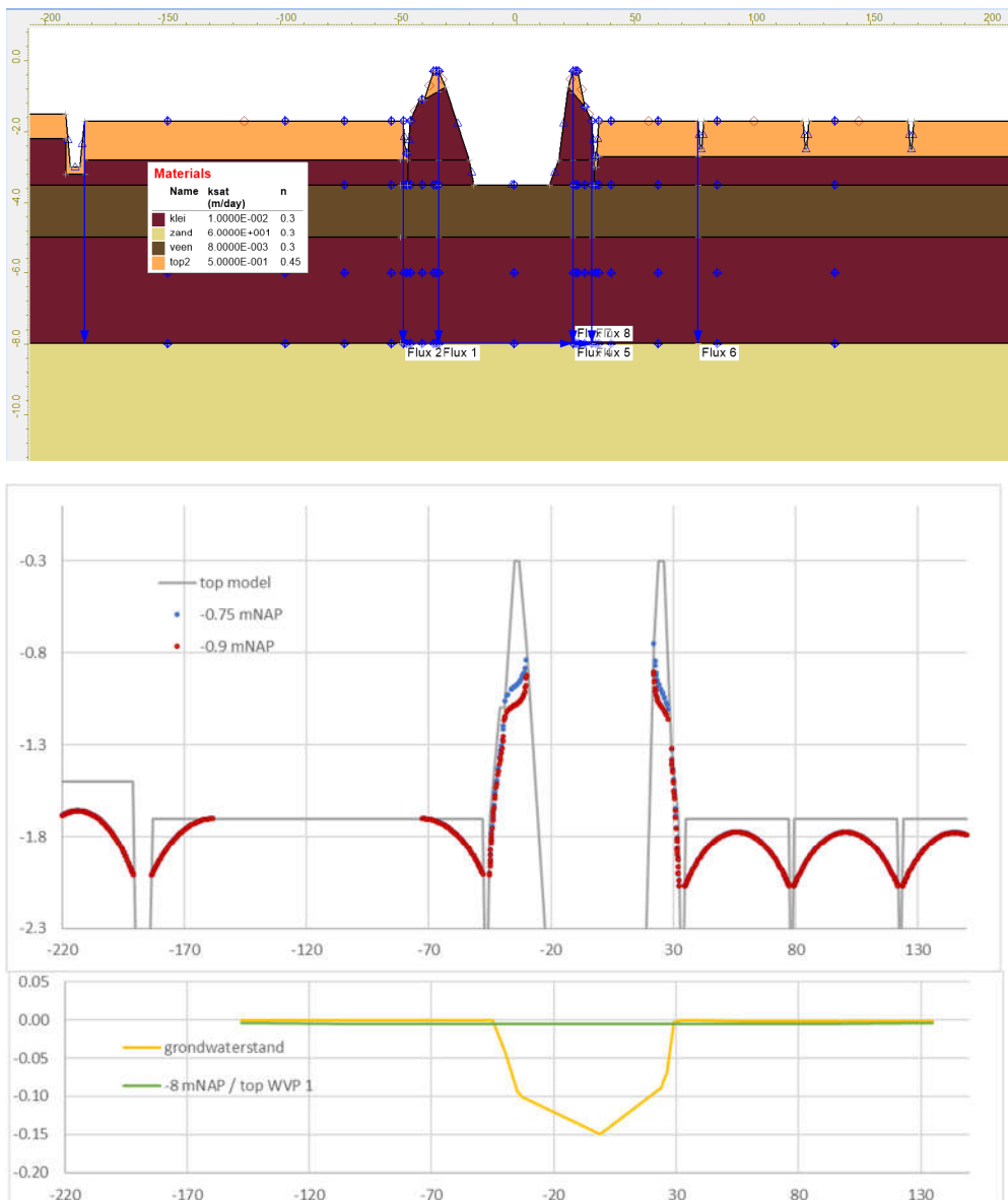
Figuur 12 Boven: Modelopzet dwarsprofiel (ingezoomd). Midden: berekende grondwaterstand (mNAP) tegen de afstand (m) voor de referentie situatie en met aangepast boezempeil. Onder: berekende effect van peilverlaging (mNAP) op twee diepten tegen de afstand (m)
