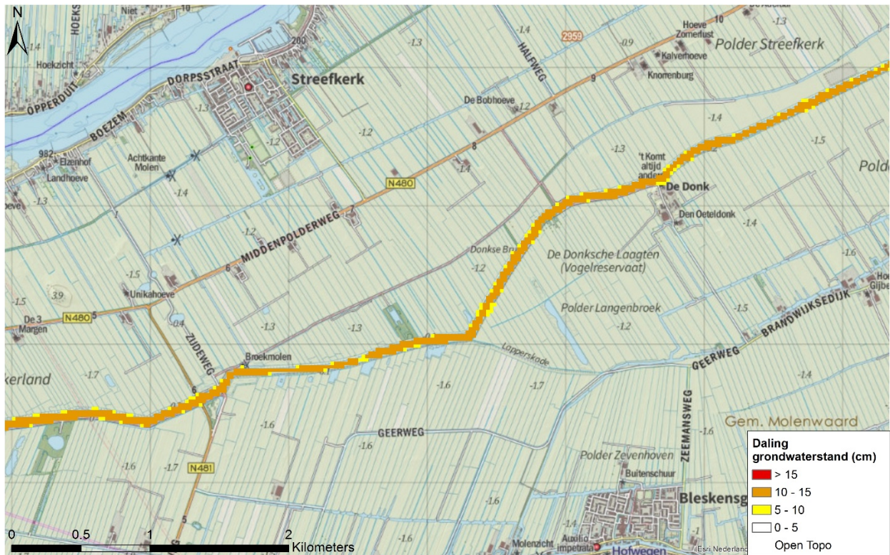
Figuur 4: Effect van peilverlaging in het Achterwaterschap op grondwaterstand in poldergebied
