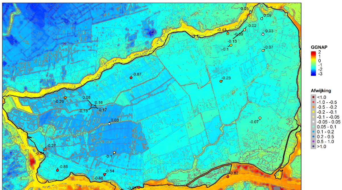
Figuur 2: Isohypsenpatroon en modelafwijkingen van het deelgebied Alblasserwaard van het MORIA-grondwatermodel. Het Achterwaterschap komt duidelijk uit het isohypsenpatroon naar voren. Hier is de grondwaterstand namelijk hoger dan in de omliggende polders.
