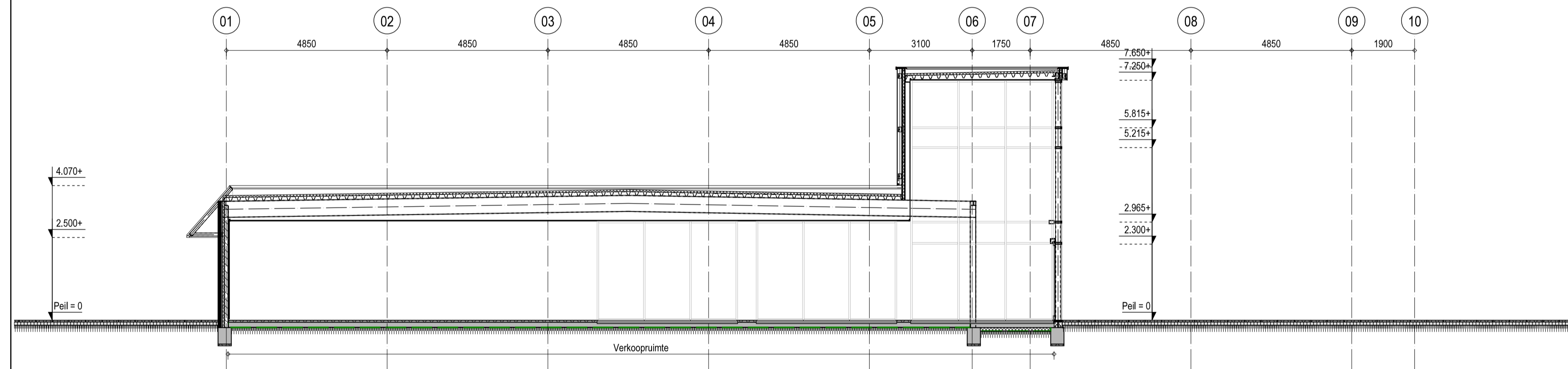
Doorsnede C-C
