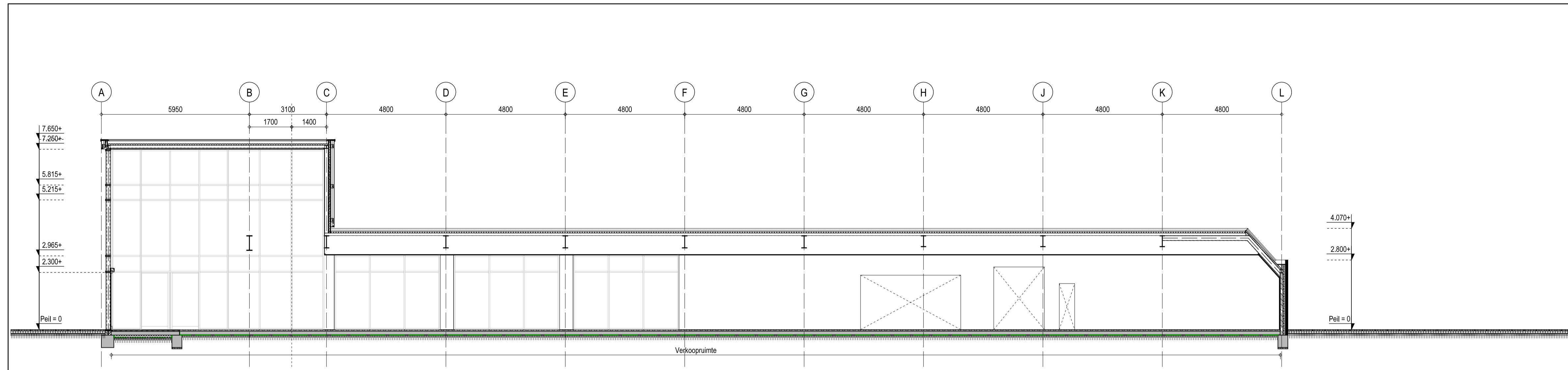
Doorsnede A-A
