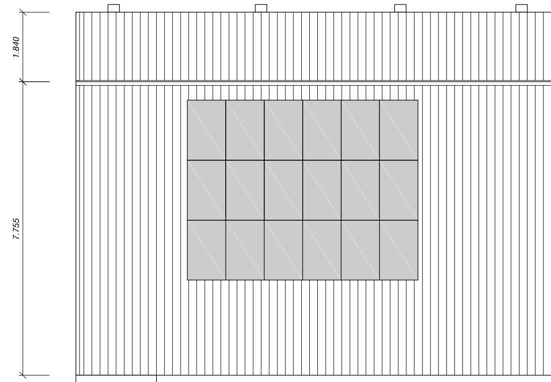
DAKAANZICHT nieuwe toestand
