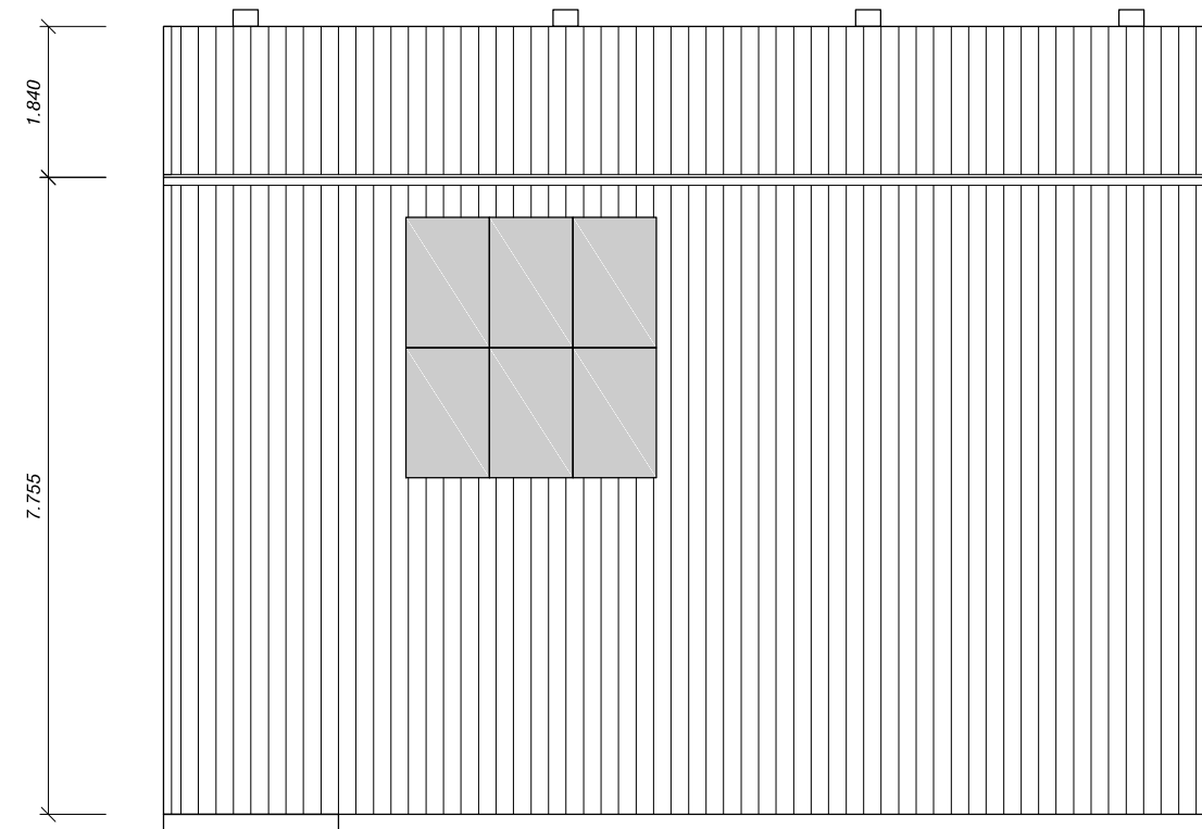
DAKAANZICHT vergunde toestand
