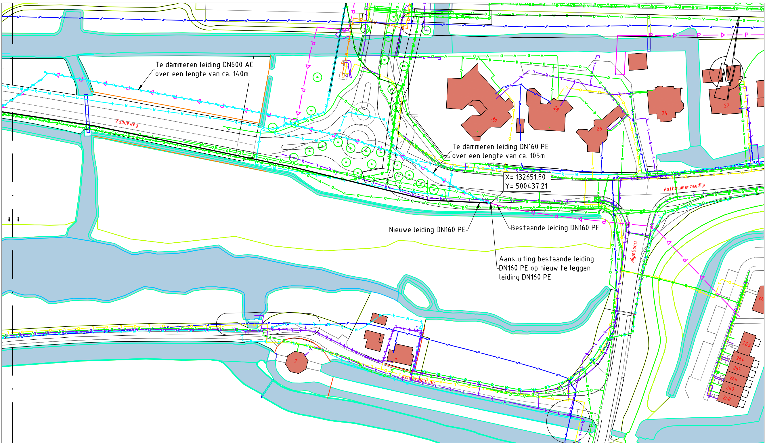
Situatie deel 2 1:1000
