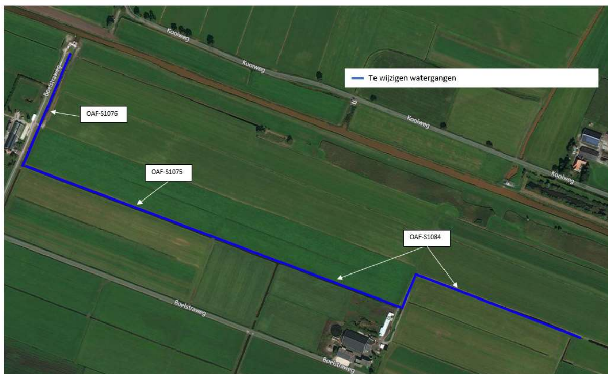
AFBEELDING 4 TE WIJZIGEN WATERGANGEN WATERSYSTEEM BOELSTRAPOLDER
