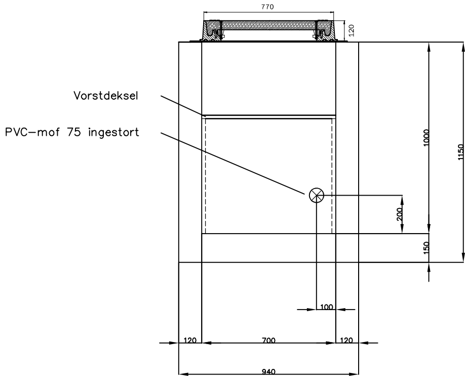
Doorsnede A-A
