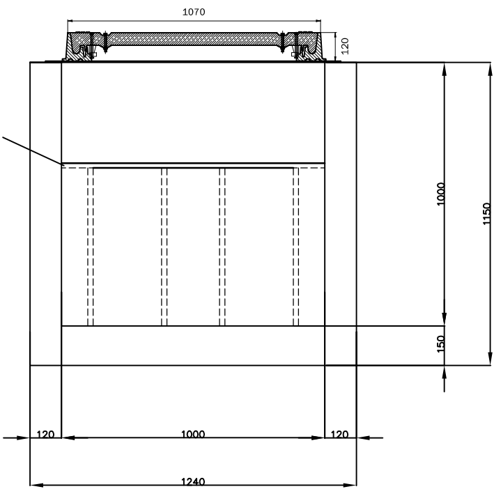
Doorsnede B-B
