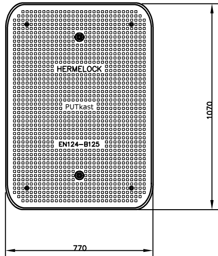
Deksel
