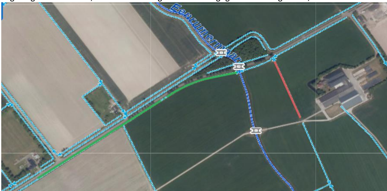
Figuur 1: Te dempen watergang weergegeven met rode lijn, te verbreden watergang weergegeven met groene lijn.
