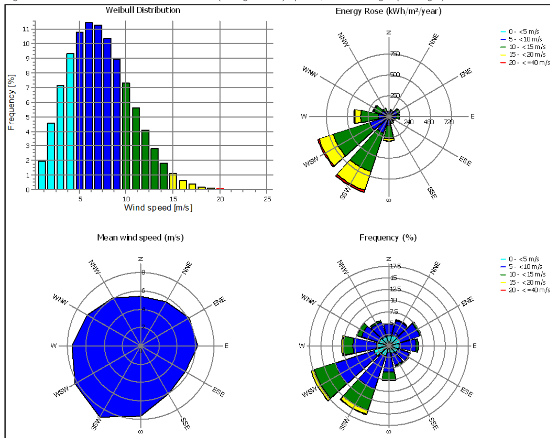
Figuur 2.1 Karakteristieken lokaal windklimaat (zoekgebied 1) op 140,0 meter hoogte (ashoogte)
