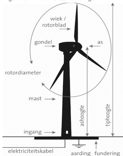
Figuur 3.1 Turbine-aanduidingen
