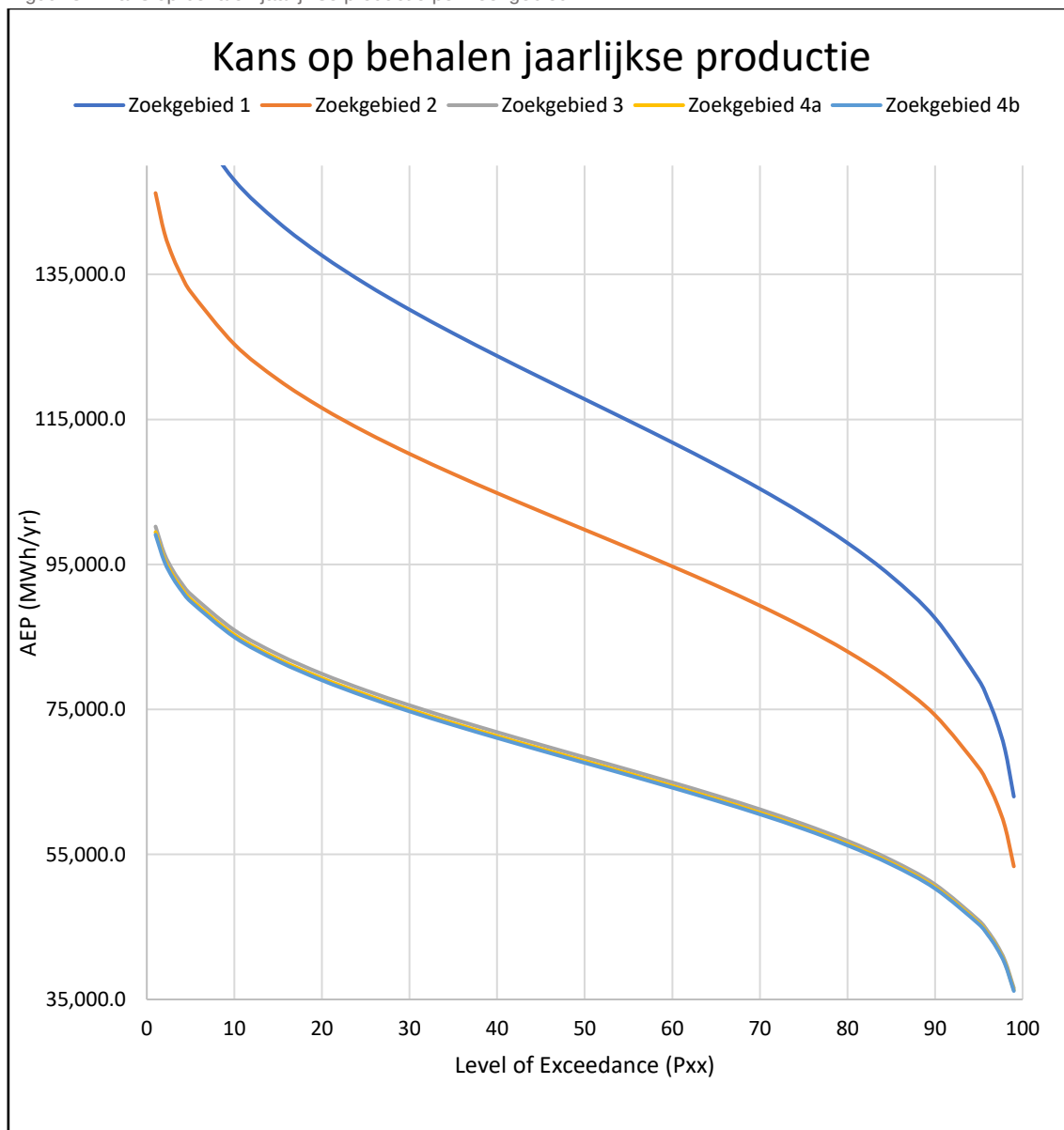
Figuur 3.1 Kans op behalen jaarlijkse productie per zoekgebied
