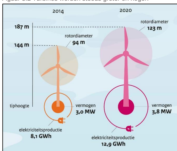
Figuur 3.2 Turbines worden steeds groter en hoger. 14
