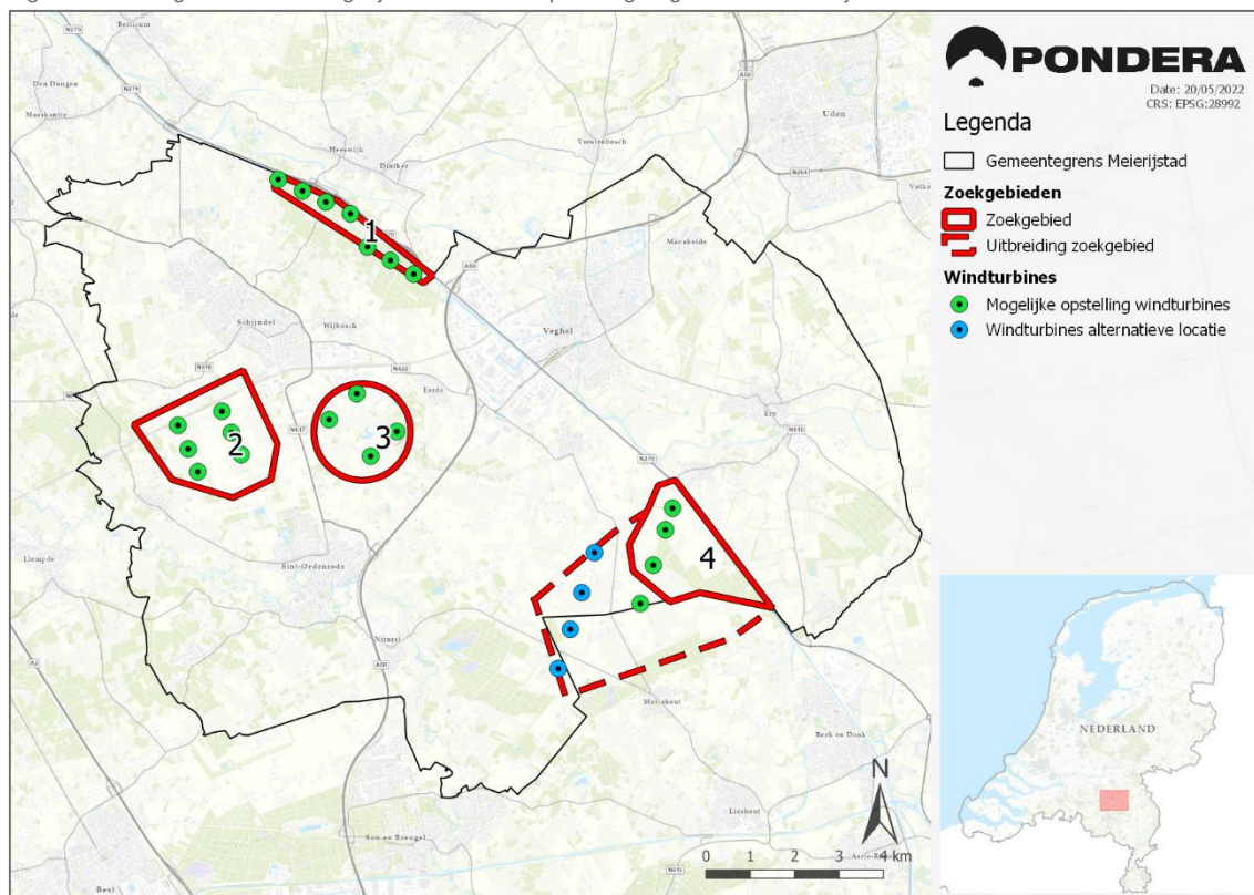
Figuur 1.1 Zoekgebieden en mogelijke windturbineopstellingen gemeente Meierijstad
