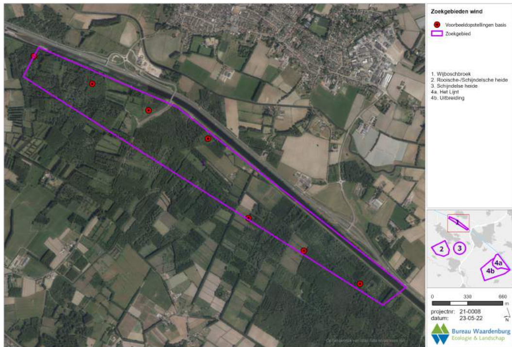
Figuur 4.1 Zoekgebied 1 - Wijboschbroek incl. mogelijke windturbinelocaties
