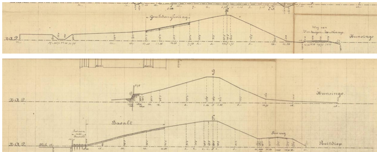
Figuur 10. Dijkprofielen Provinciale dijk tussen Zoutkamp en Panseerpolder (boven) en Afsluitdijk langs het Reitdiep (onder).1916. GA, nr. 817_3992.11.
