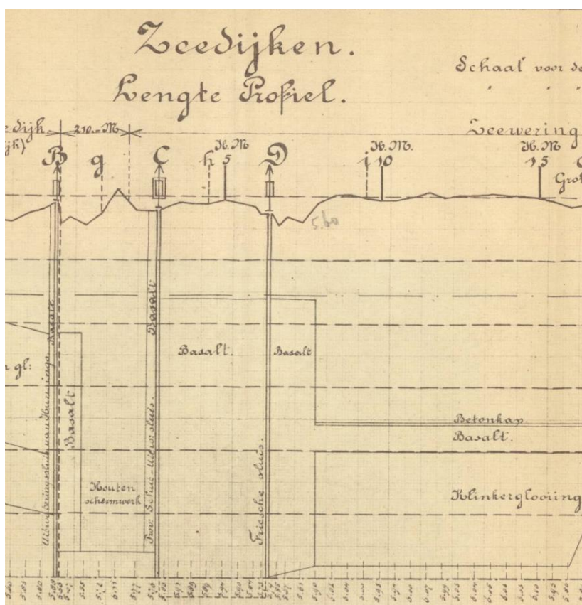
Figuur 11. Dijkprofielen Provinciale dijk tussen Zoutkamp en Panseerpolder en Afsluitdijk langs het Reitdiep.1916. B. Hunsingosluis, C. Reitdiepsluis. GA, nr. 817_3992.11
