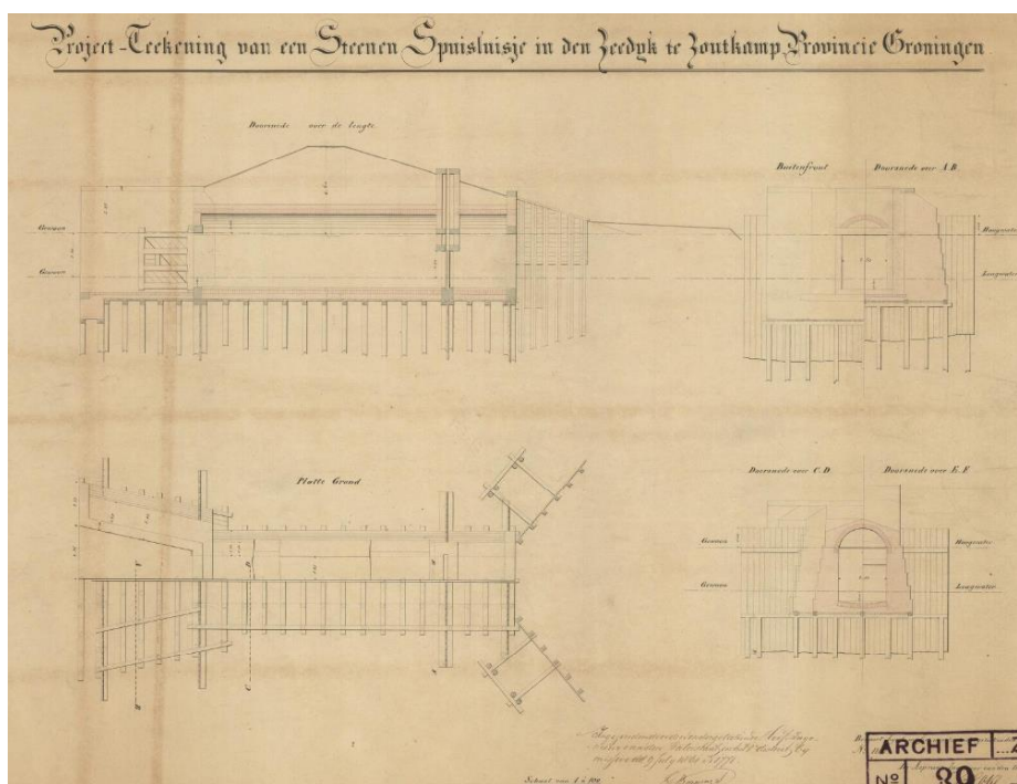
Figuur 28. Ontwerp van een stenen spuisluize in de dijk bij de haven, 1861. Bron: GA, nr. 817_3102.5.
