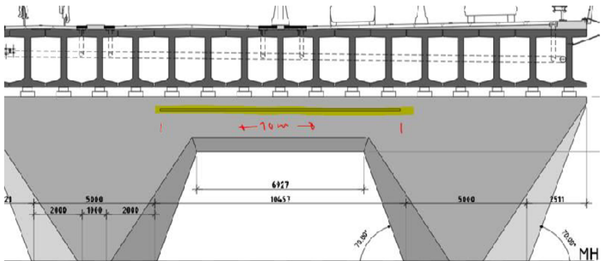
Afbeelding 2. Locatie van de te plaatsen kunstmatige nesten voor de huiswaluw (geel) op een pijler. Dit wordt op 2 pijlers toegepast. Zodat er in totaal 44 nestkasten worden geplaatst met ruimte ertussen waar huiswaluwen zelfstandig nieuwe nesten kunnen maken. Er wordt hiermee ruimte geboden aan ruim 44 huiswaluwen.
