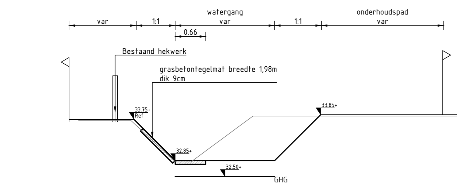
Dwarsprofiel A-A Schaal 1:50
