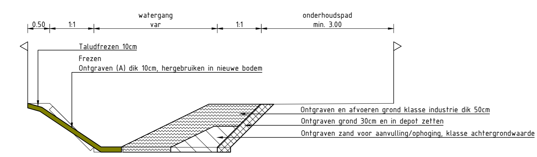
Principe ontgravingsprofiel Schaal 1:50
