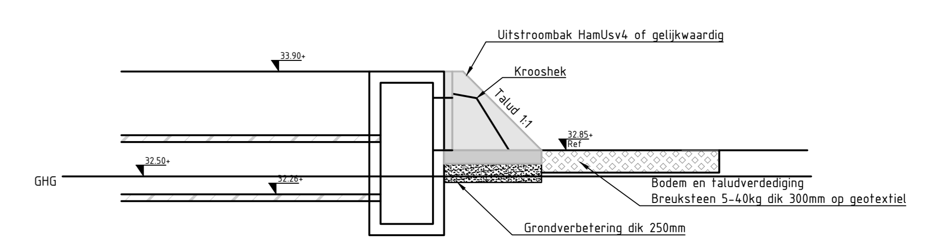
Principedetail uitstroombereiding Schaal 1:50
