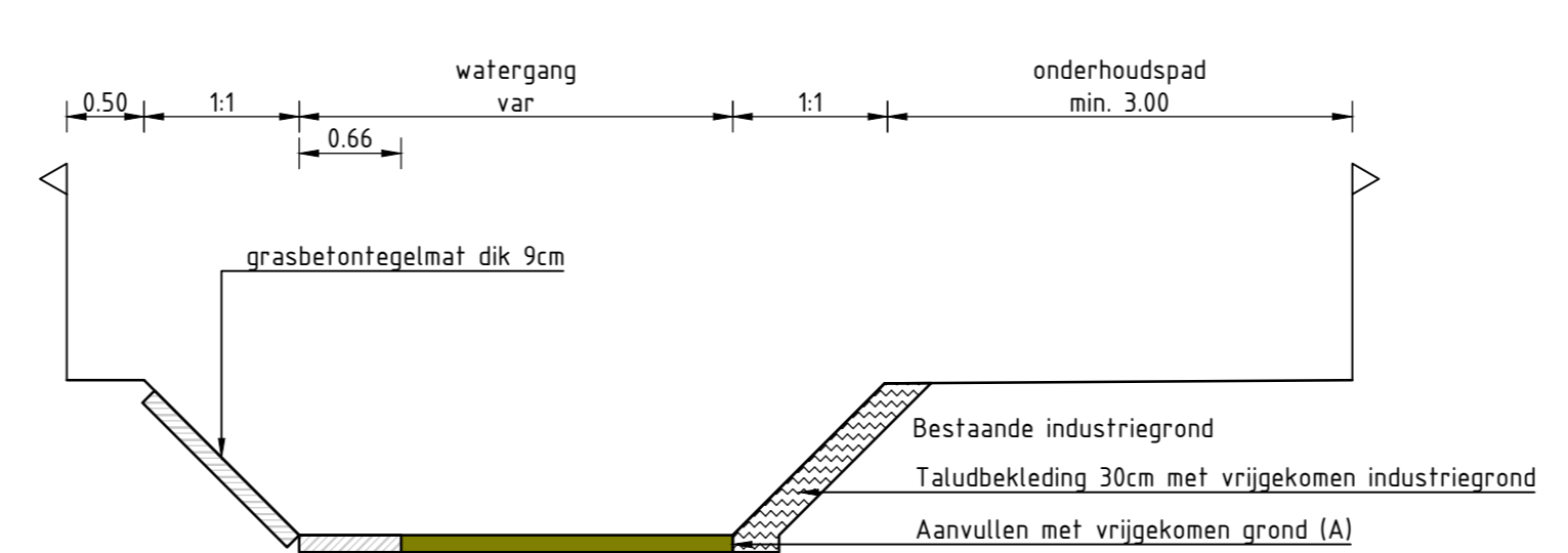
Principe aanvullingsprofiel Schaal 1:50
