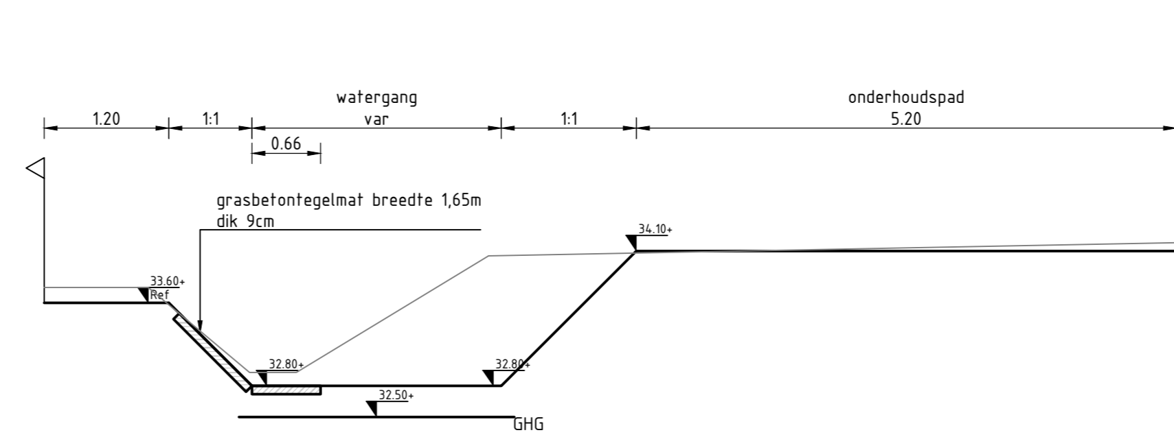
Dwarsprofiel C-C Schaal 1:50
