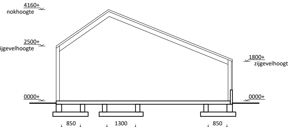
doorsnede B-B
