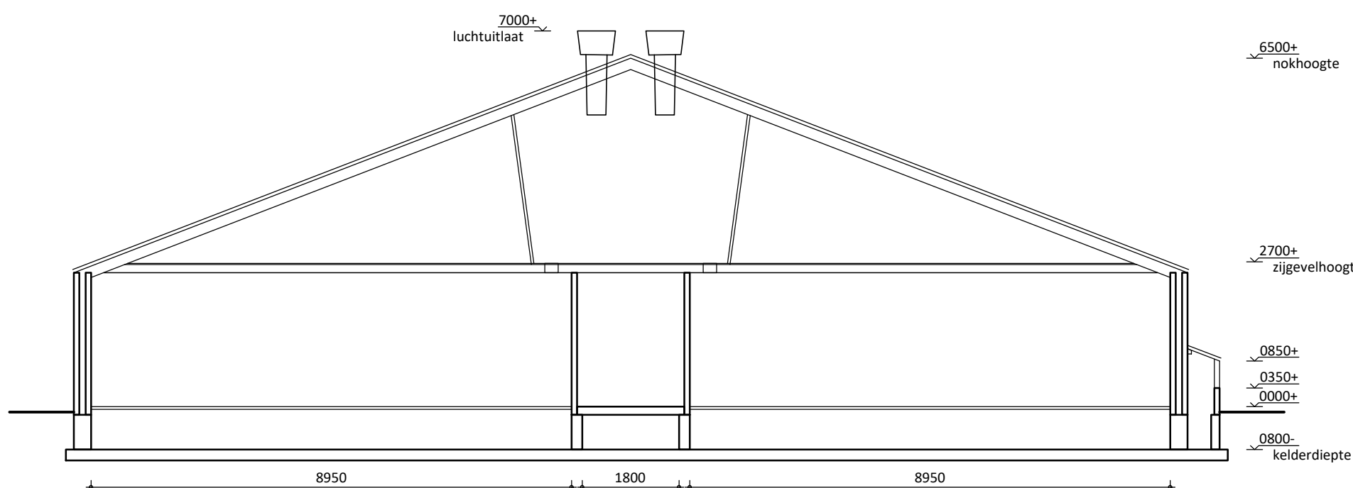
doorsnede L-L
