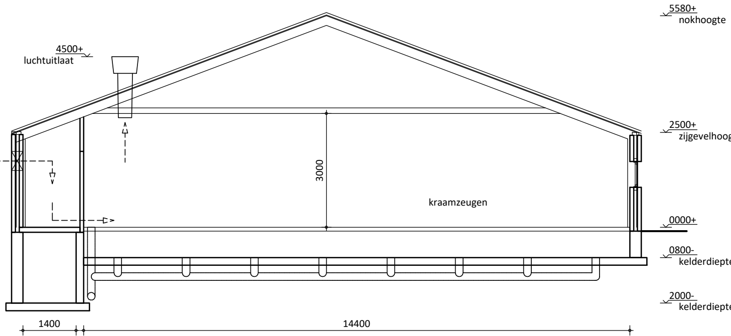
doorsnede G-G
