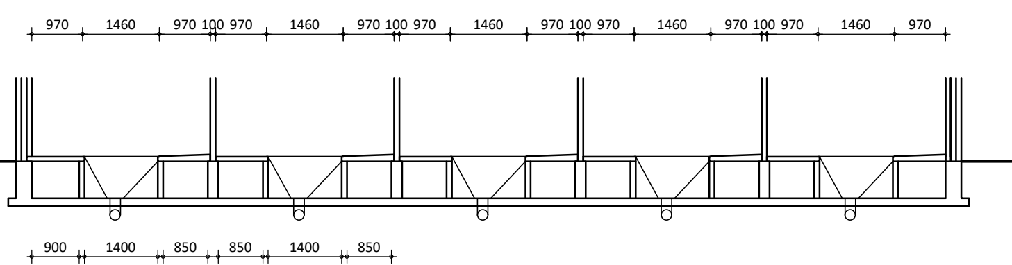
doorsnede G - G
