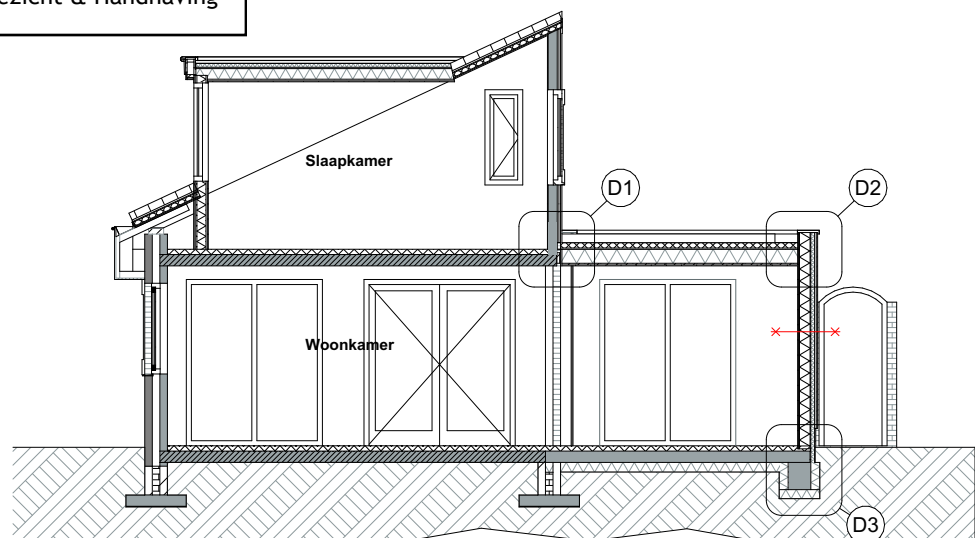
Doorsnede B-B
