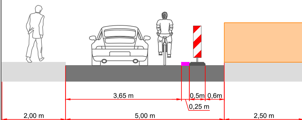
Dwarsdoorsnede A-A
