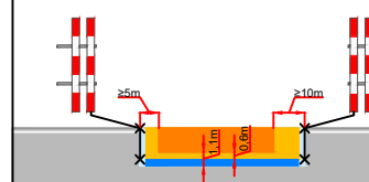
Werkvakindeling ETW
