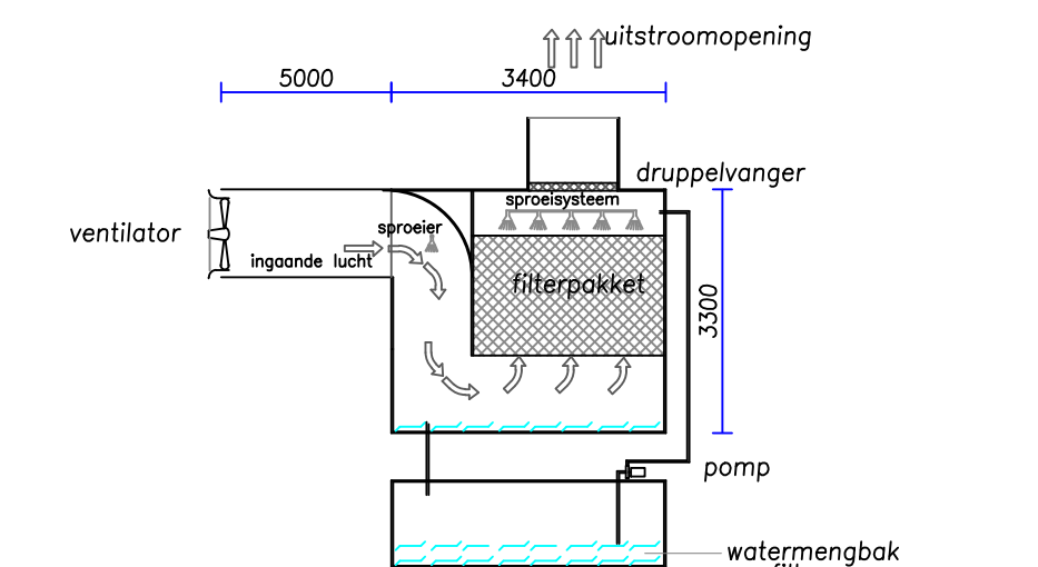
Schema biologisch combi-luchtwater : BWL 2009.12.V4 circulatiepomp voorzien van urenteller spuiwatermeting d.m.v. geijkte waterpulsometer
