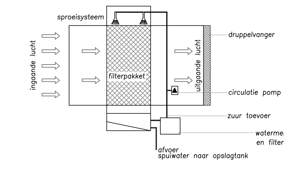
Schema chemisch luchtwater : BWL 2008.09.V6 chemisch luchtwatersysteem 95% ammoniakemissiereductie, voor kraamzeugen, gesp. biggen, guste en dragende zeugen, dekberen en (inclusief opfokberen en opfokzeugen) Zie systeembeschrijving April 2009
