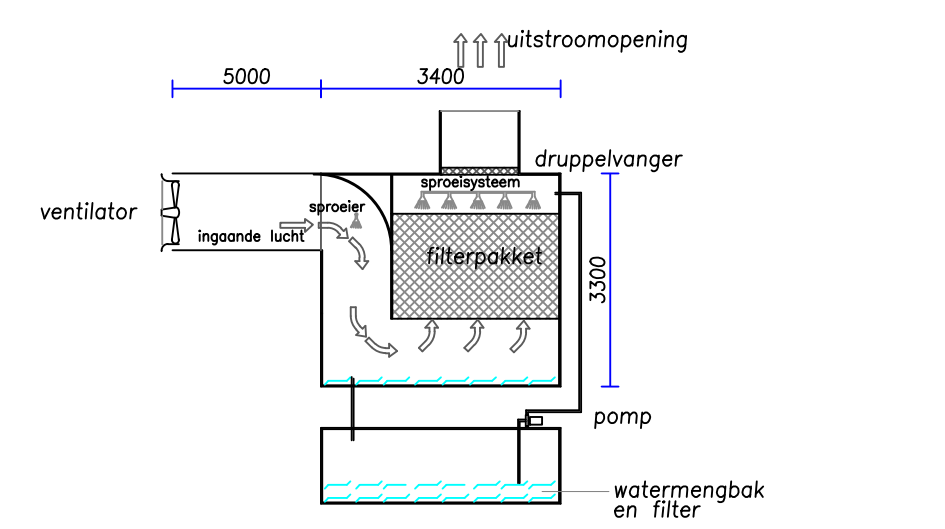
Schema biologisch combi-wat/wasser : BWL 2009.12.V1 / BWL 2009.12.V4
