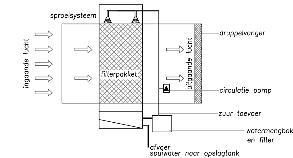
Schema chemisch luchtwater : BWL 2008.09.V1 chemisch luchtwaterstelsel 555 amoniamreductie voor kraanwater, gres, liggen, gulle en droppende zeugen, debeken en vleesvarkens (inclusief oplosbare en oplosbare) Zie systeembeschrijving April 2009
