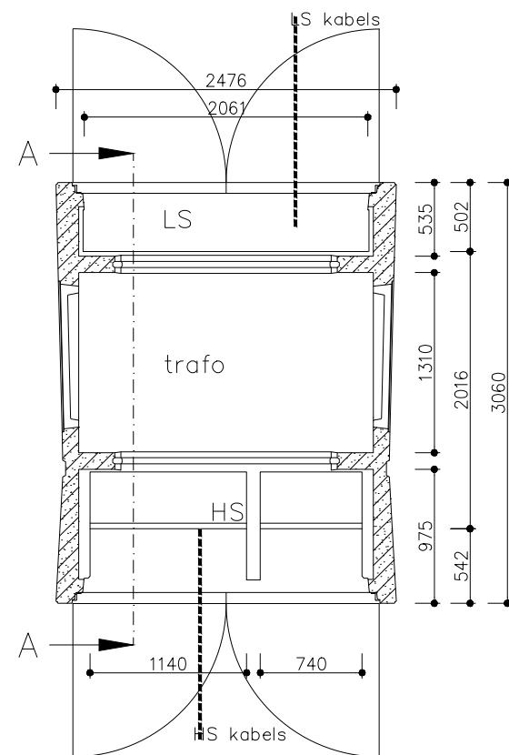
PLATTEGROND
