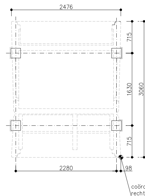
PALENPLAN
