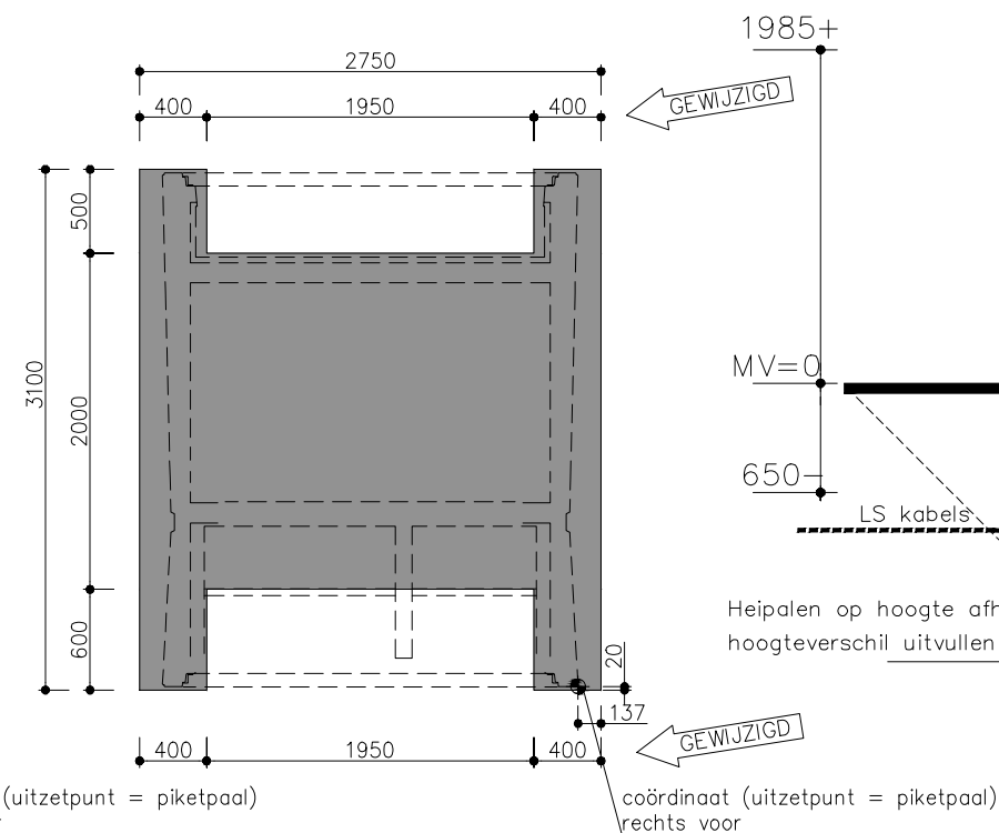
FUNDERING GESTABILISEERD ZAND
