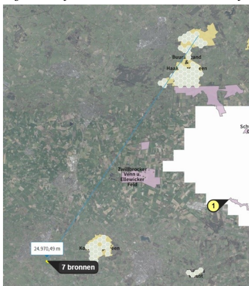
Figuur 2: afstand tussen bron en dichtstbijzijnde hexagoon waar een toename plaatsvindt in AERIUS Calculator.
