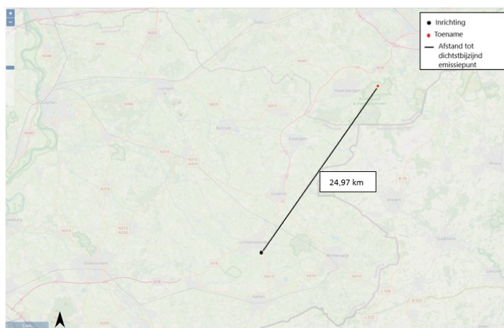
Figuur 1: afstand tussen bron en dichtstbijzijnde hexagoon waar een toename plaatsvindt.
