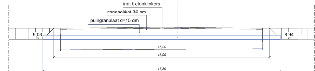
lengteprofiel 2 schaal 1 : 100
