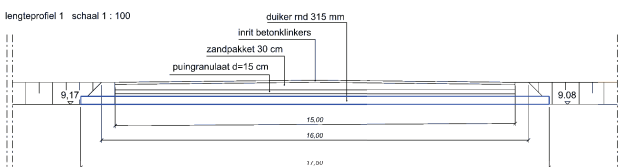
lengteprofiel 1 schaal 1 : 100
