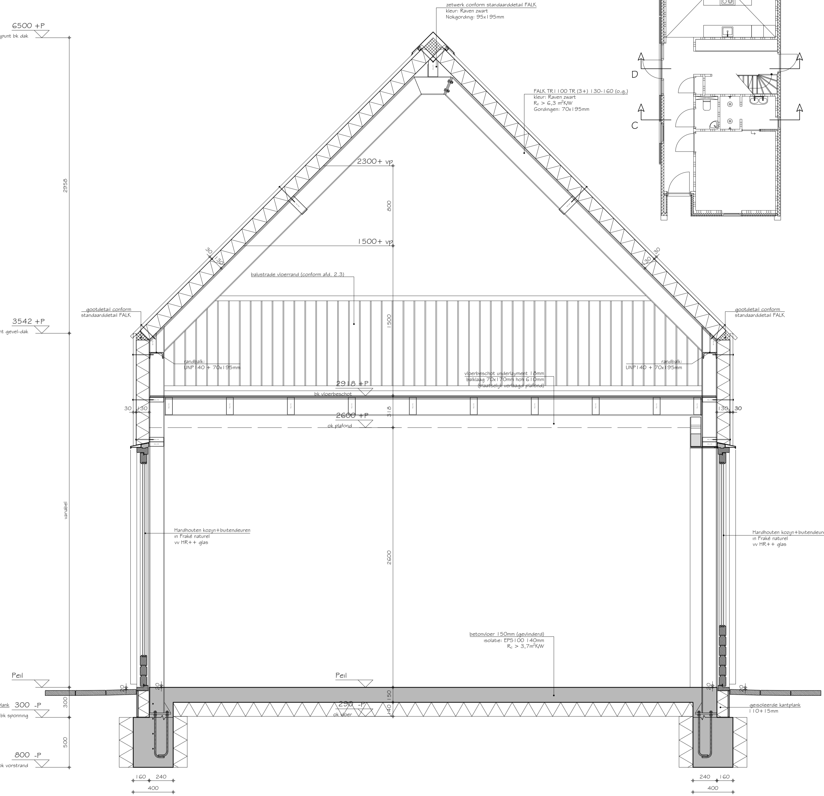
DOORSNED E D-D
