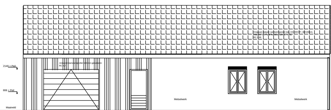
Achtergevel nieuw
