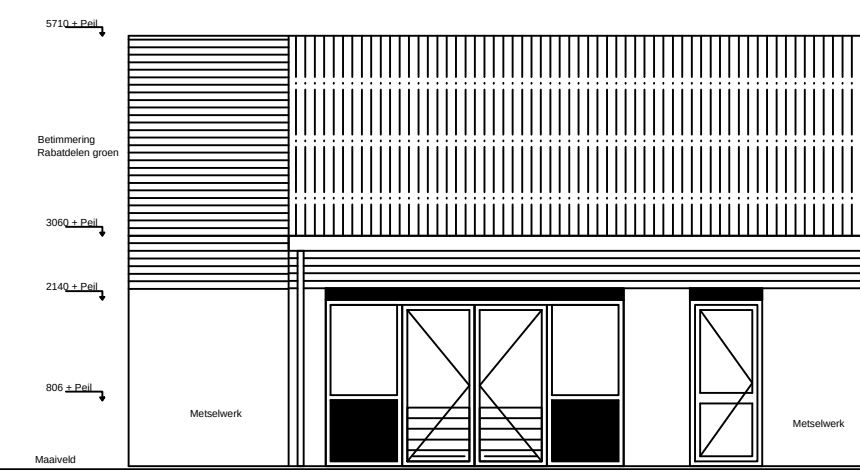
Voorgevel bestaand
