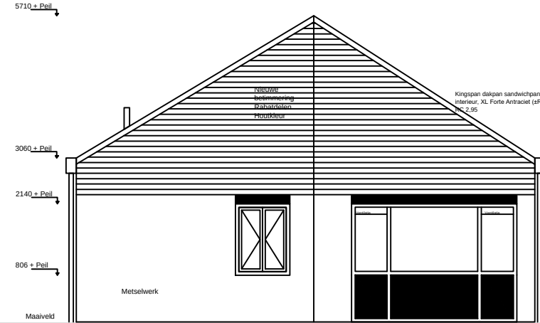
Rechter zijgevel nieuw
