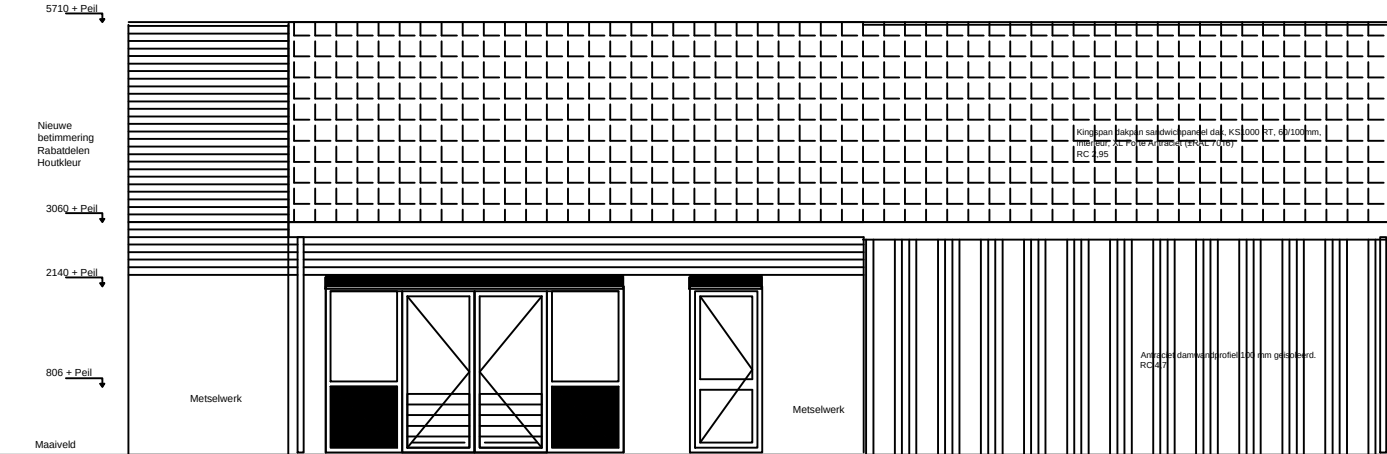
Voorgevel nieuw
