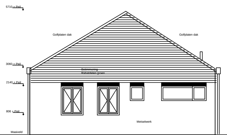
Linker zijgevel bestaand
