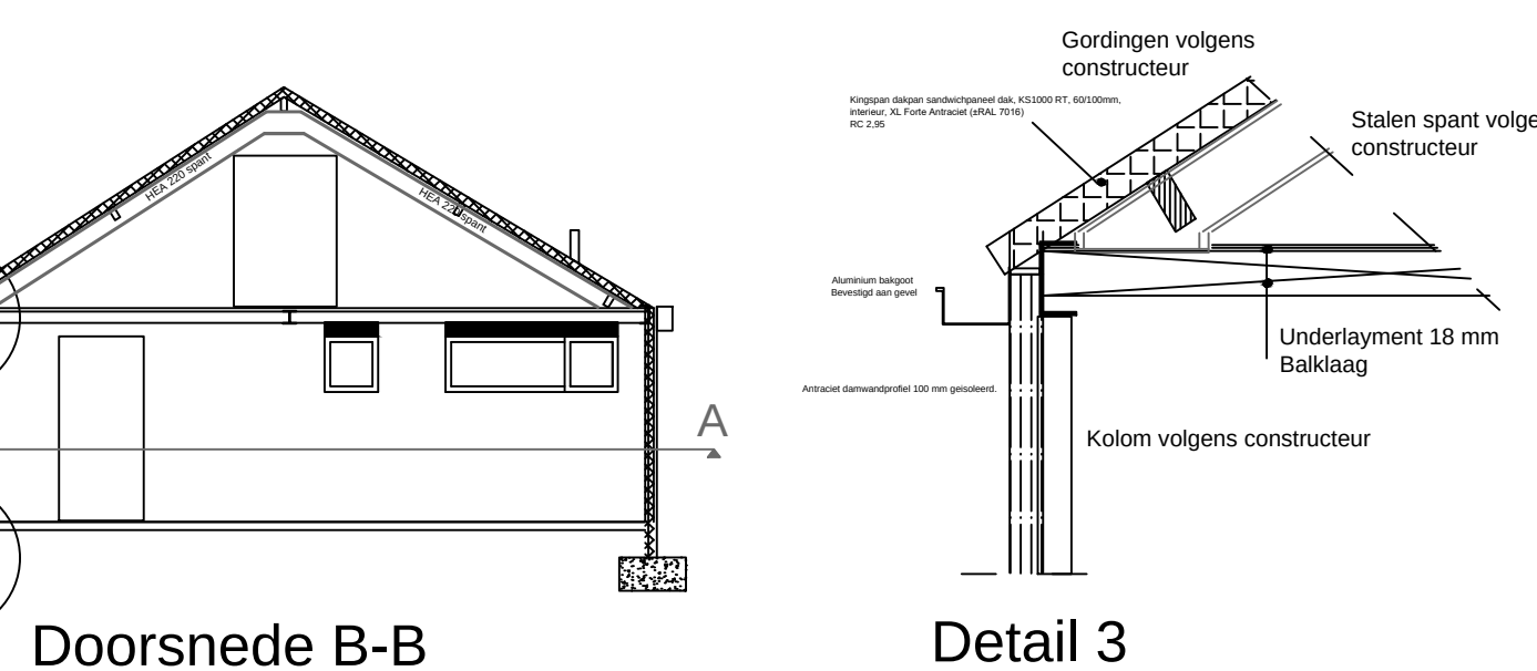
Doorsnede B-B
