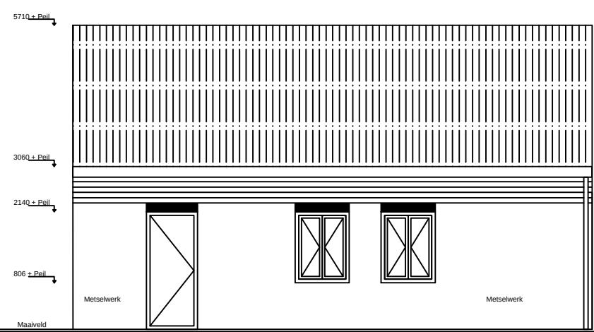
Achtergevel bestaand
