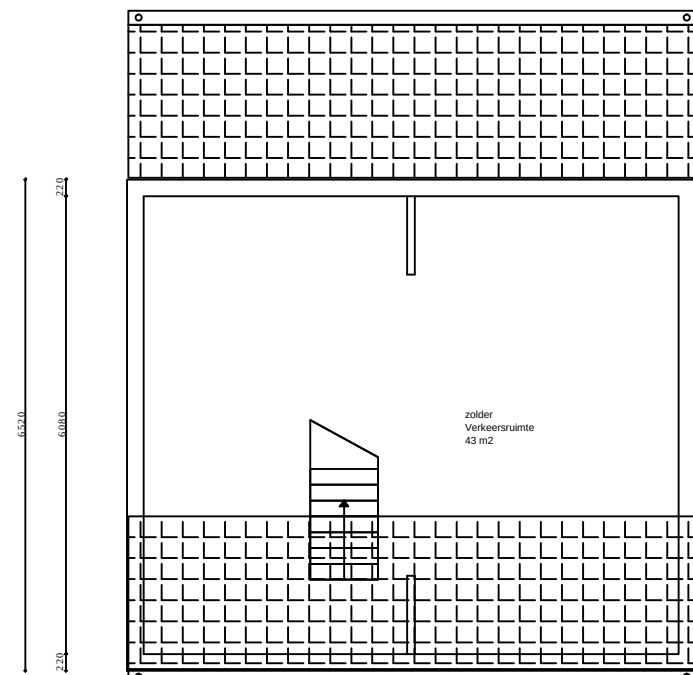
Zolder bestaand
