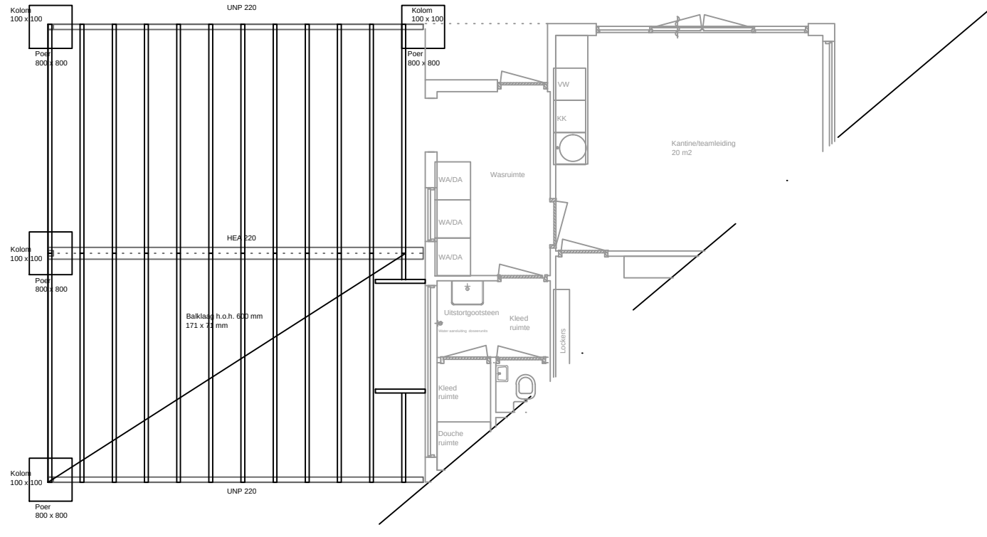
Constructie OPZET
