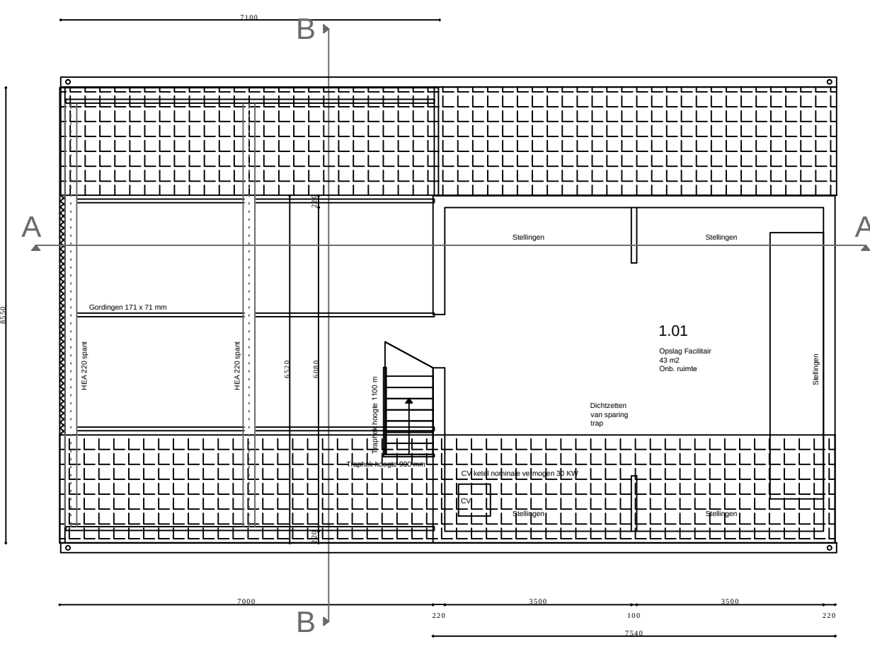
Zolder nieuw
