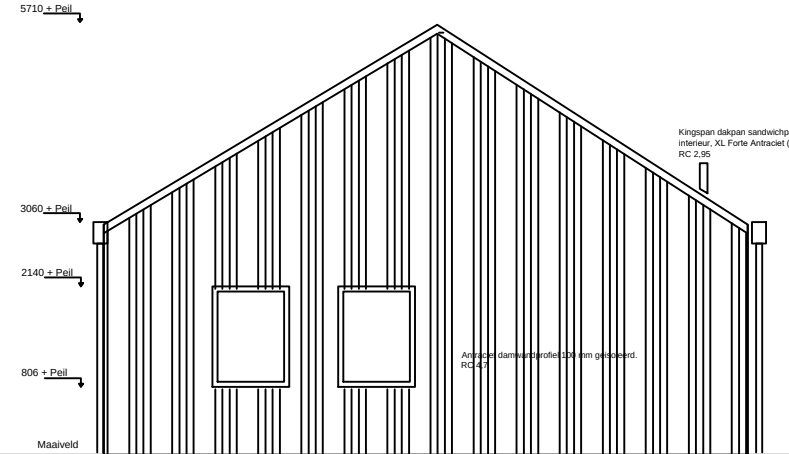
Linker zijgevel nieuw
