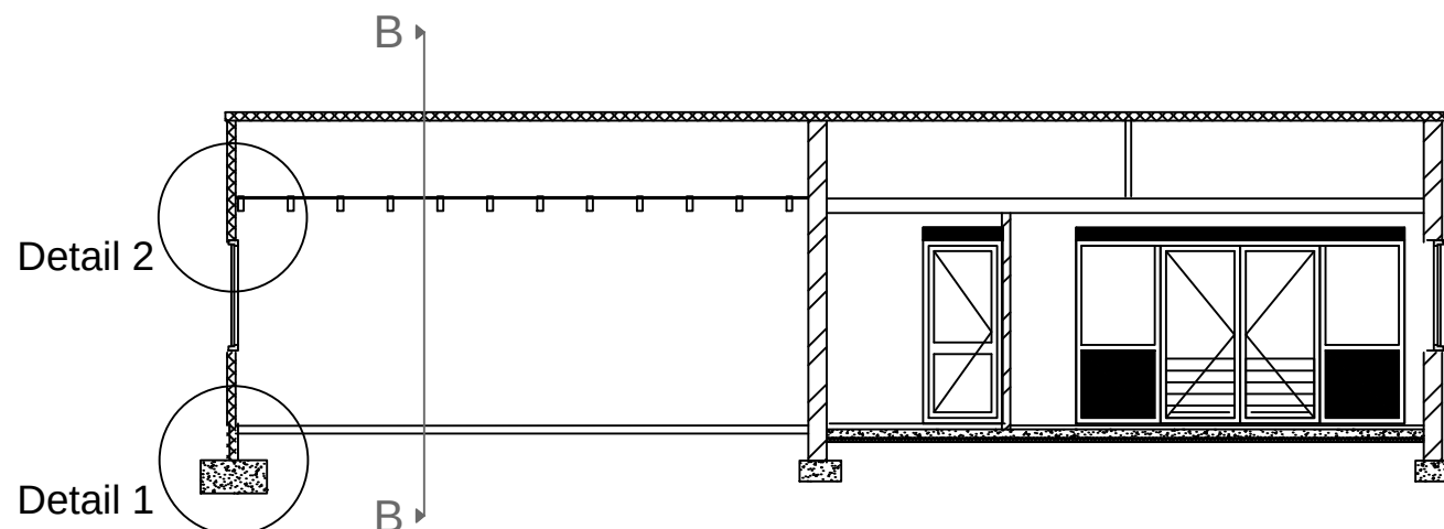
Doorsnede A-A
