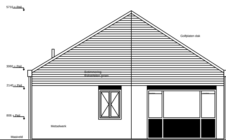
Rechter zijgevel bestaand
