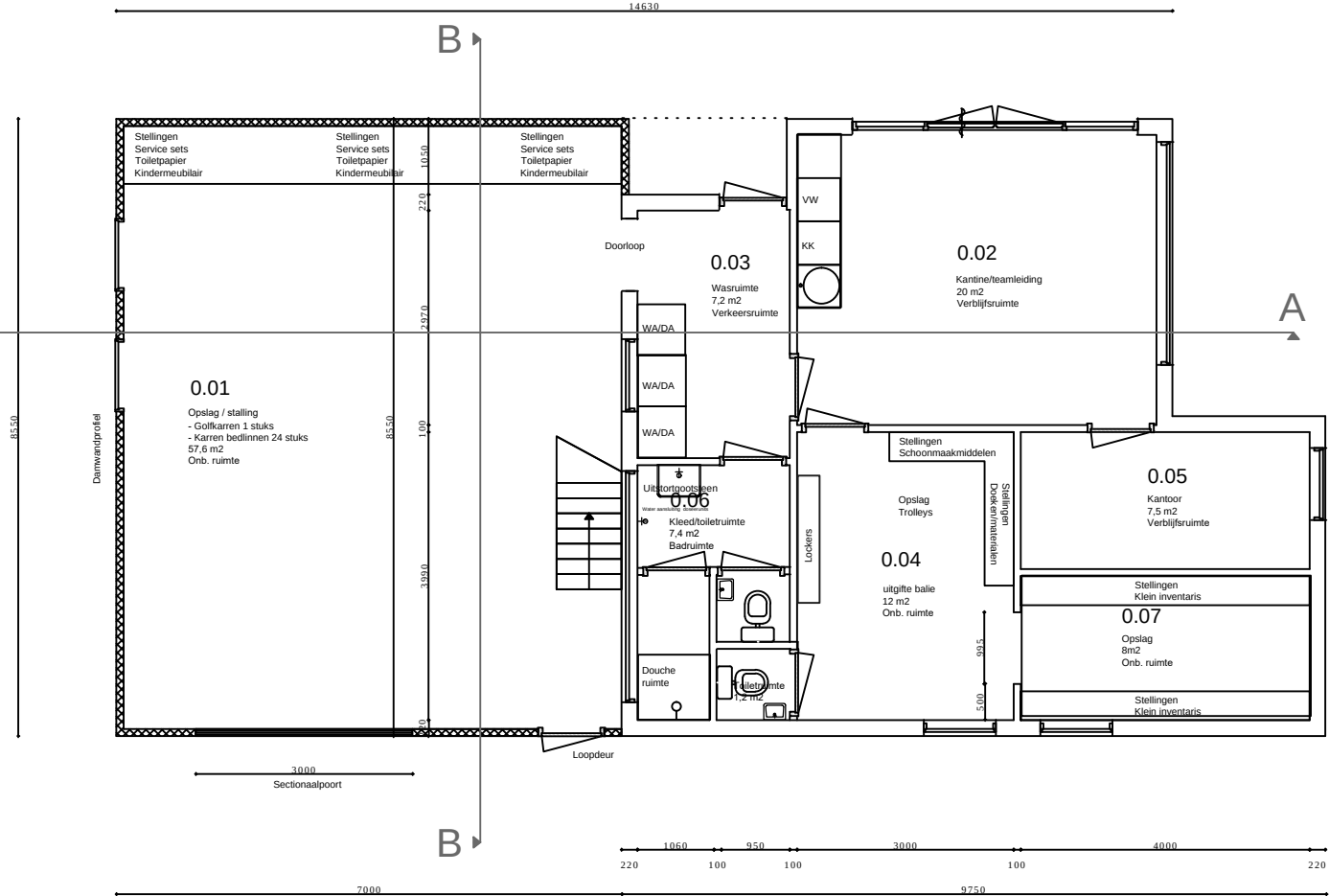
Begane grond nieuw
