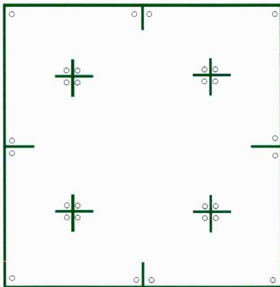
Figuur 5.1 Principe voor het plaatsen van het raster (vangkruizen) en vangemmers
