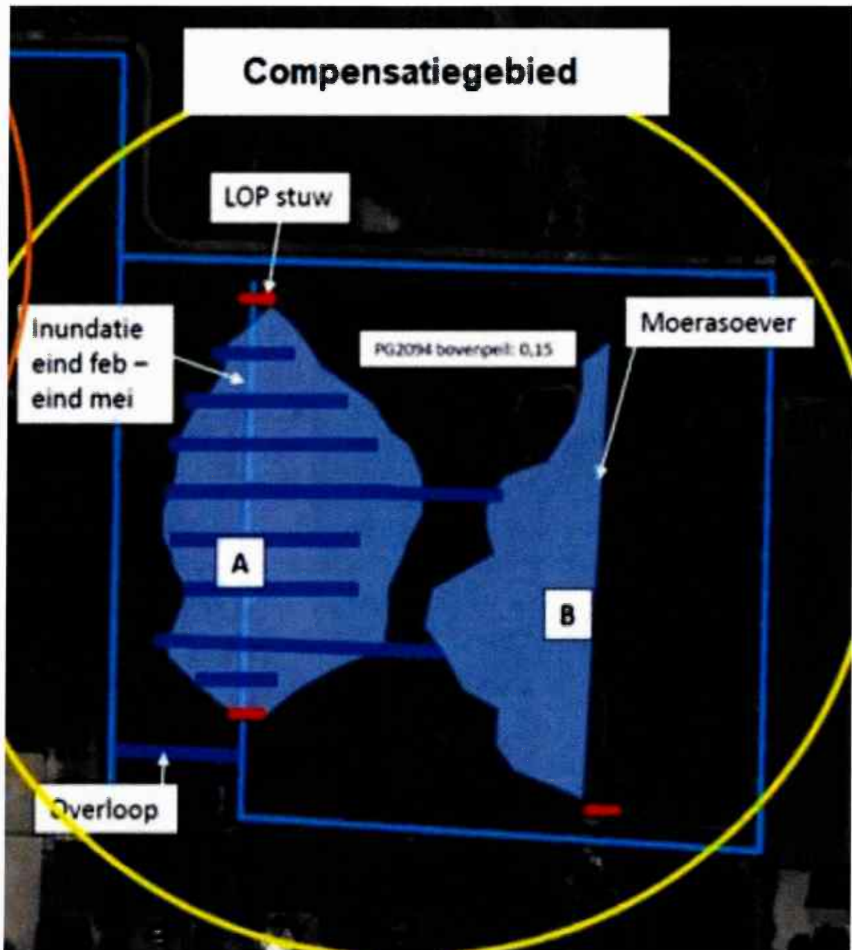
Figuur 2.4 Schetsontwerp compensatiegebied met nieuw aan te leggen moerassloten en plas-dras zones.
