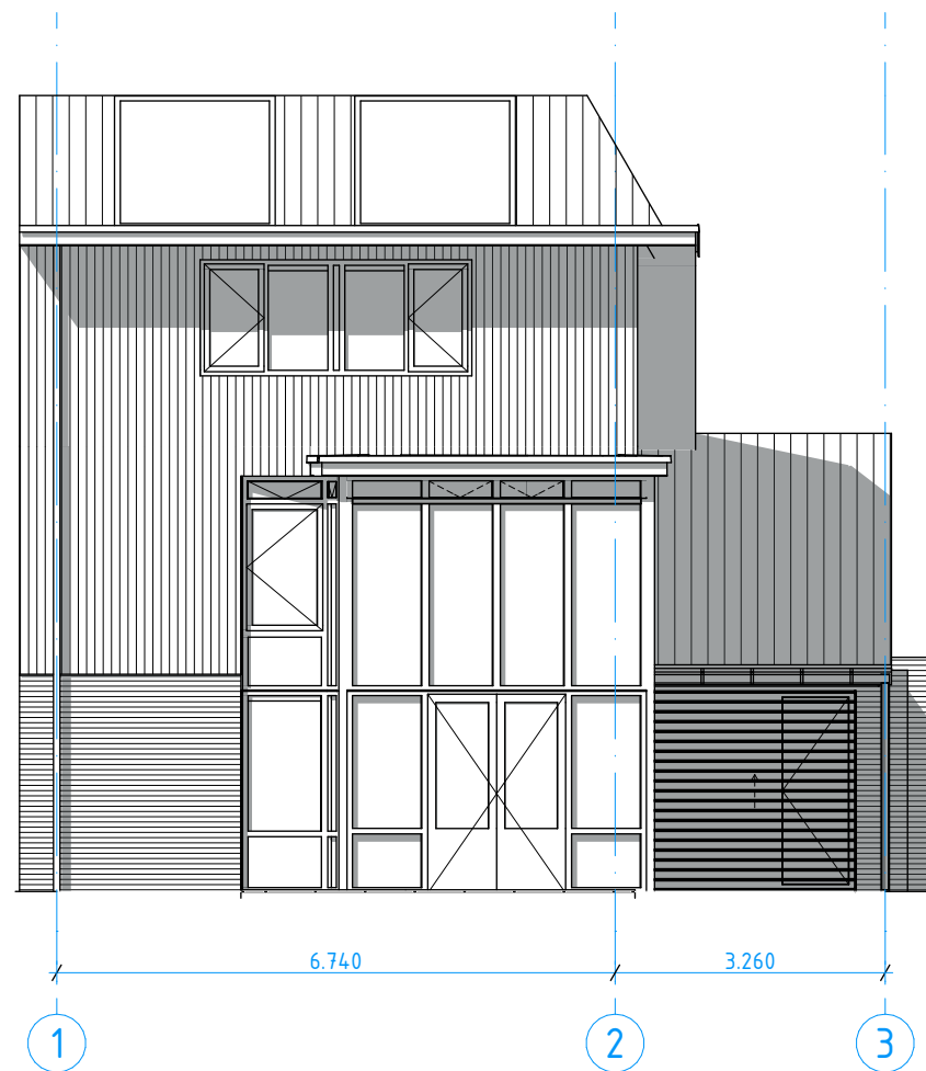
Voorgevel
