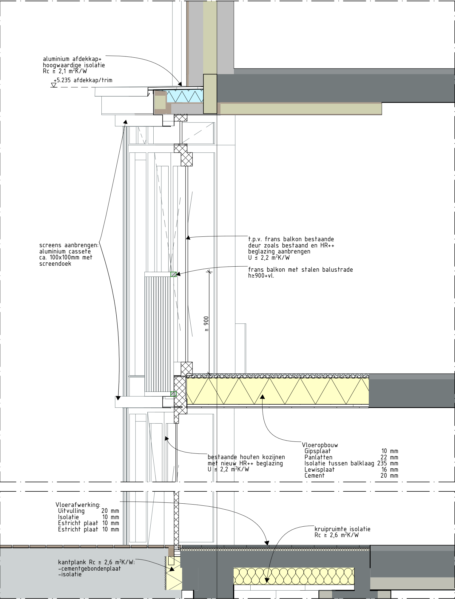
Fragment doorsnede C-C (voorgevel)
