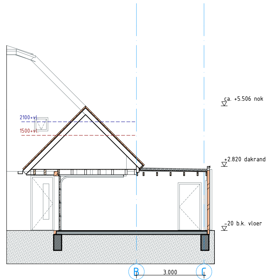
Doorsnede B-B
