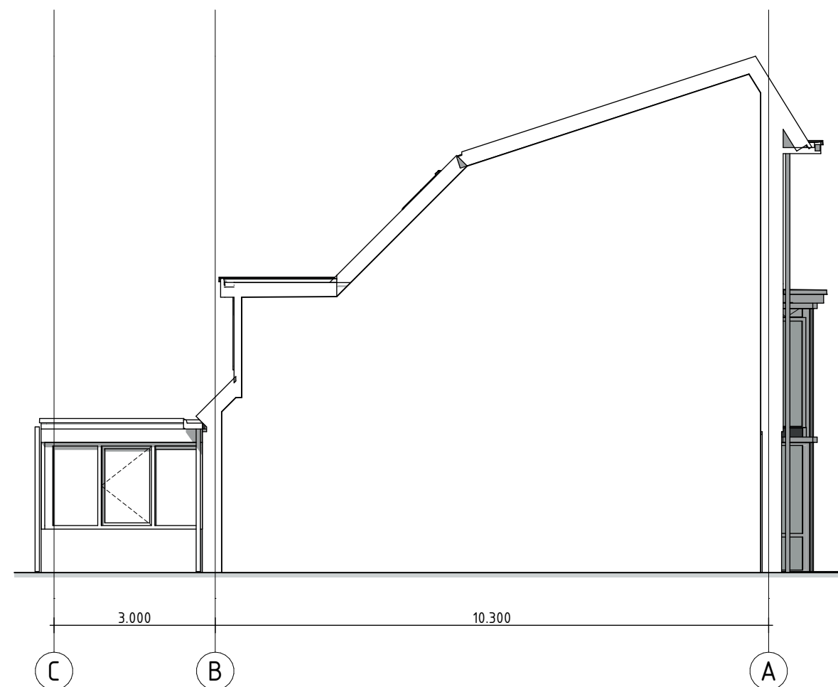
Linkergevel
