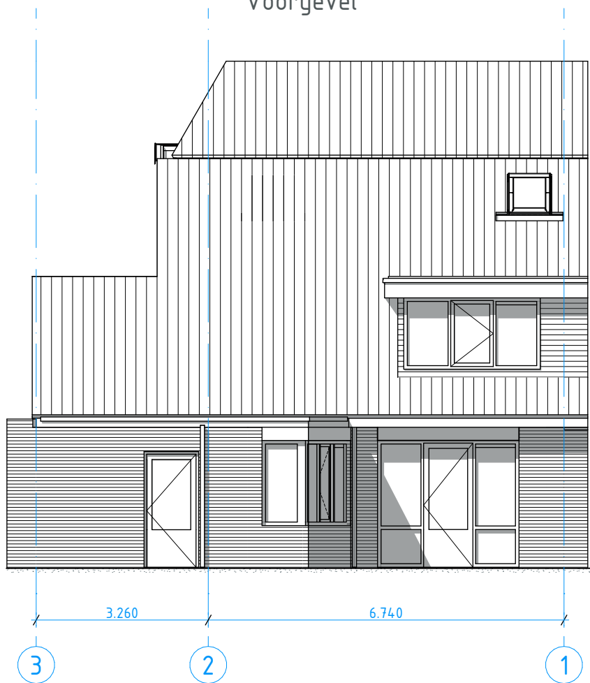
Achtergevel
