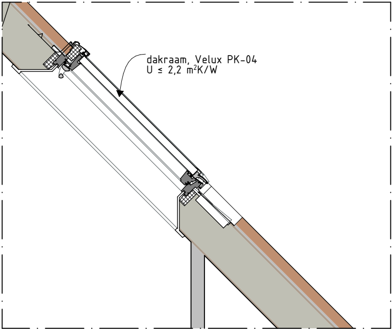
Fragment doorsnede C-C (dakraam)
