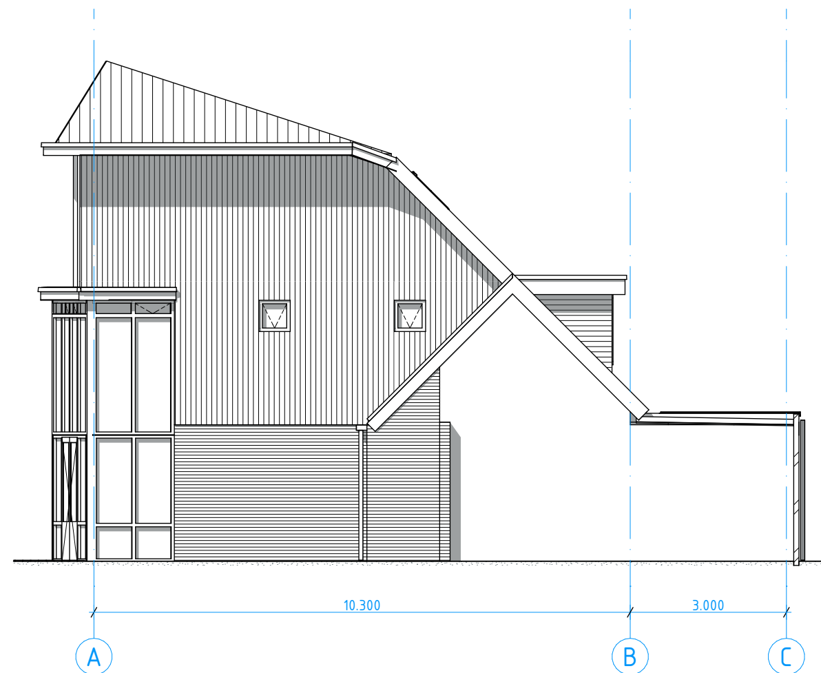
Rechtergevel
