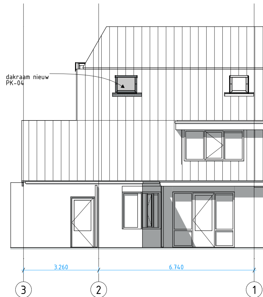
Achtergevel
