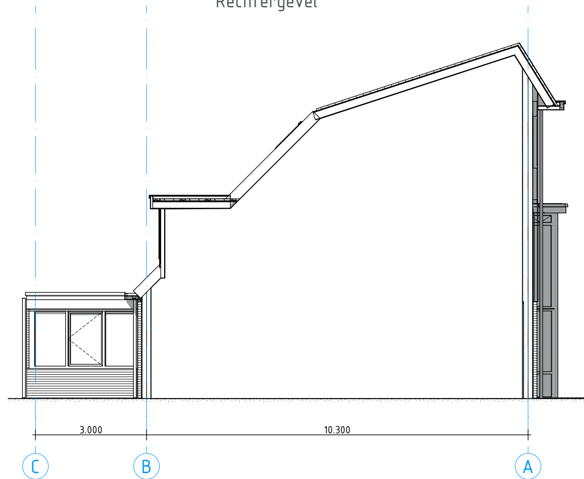
Linkergevel
