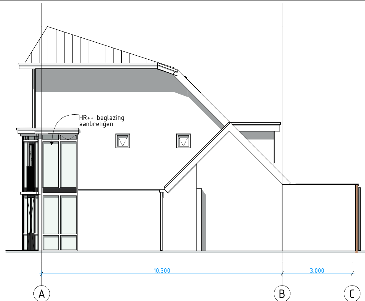
Rechtergevel
