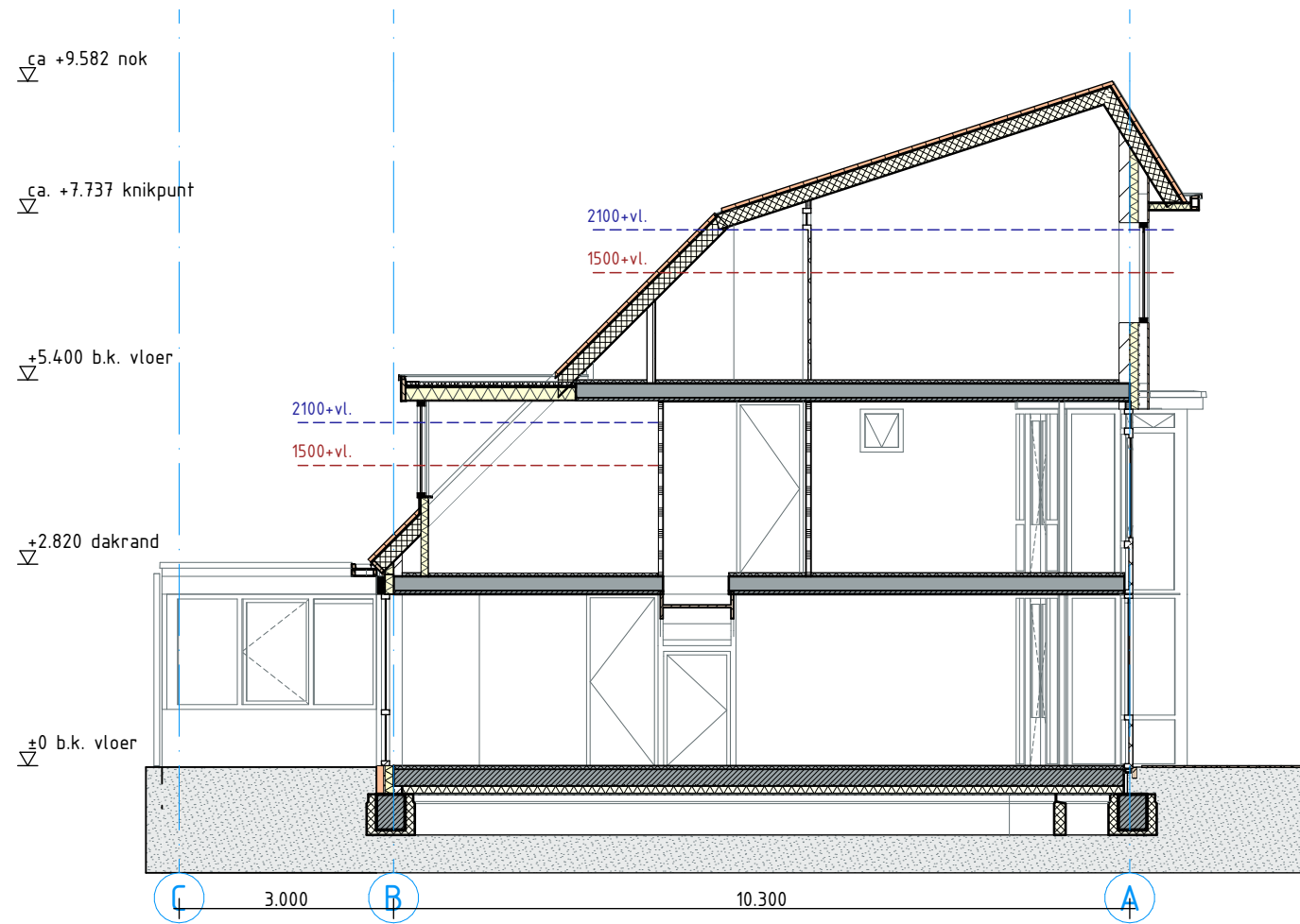
Doorsnede A-A
