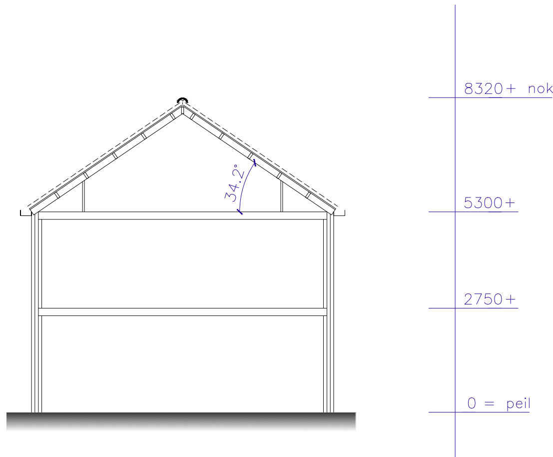
DOORSNEDE BESTAAND
