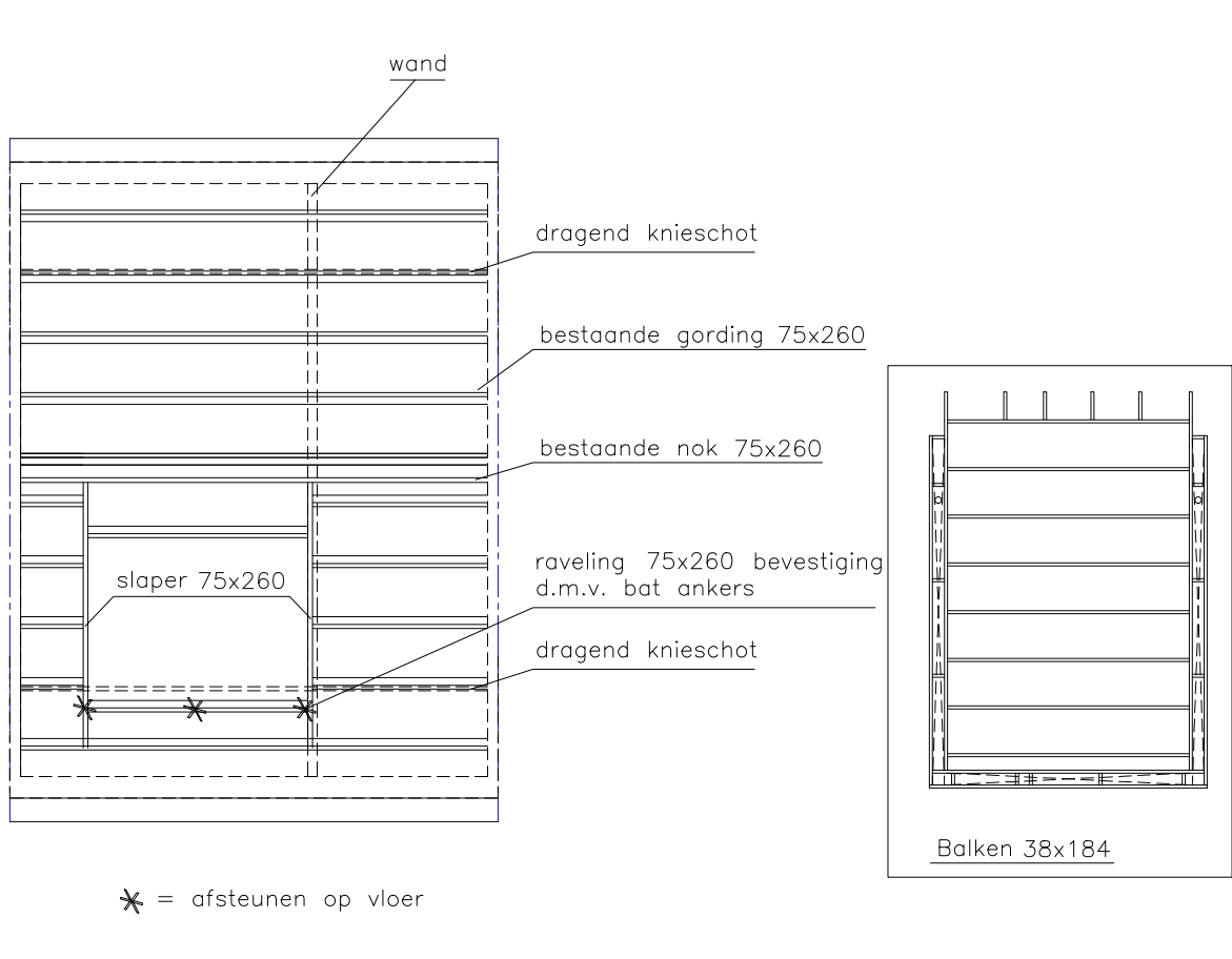
KAPPLAN NIEUW
