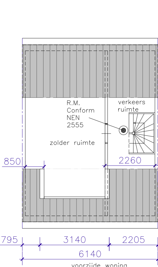
INDELING NIEUW
