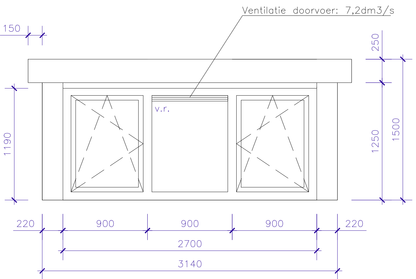
AANZICHT DAKKAPEL VOERGEVEL
