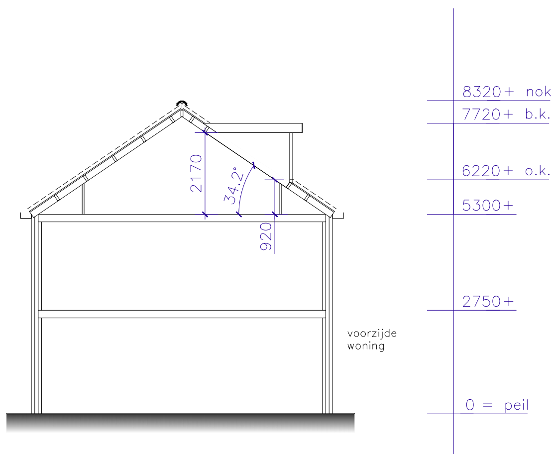
DOORSNEDE NIEUW
