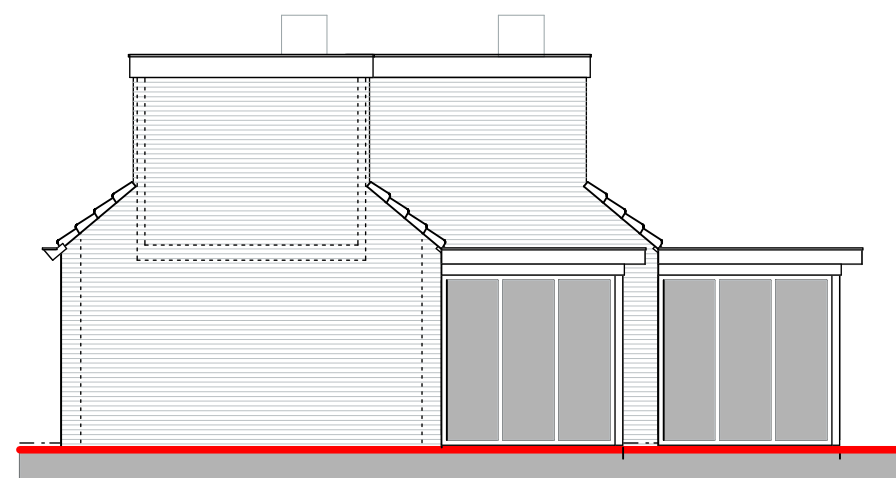
linker zijgevel
