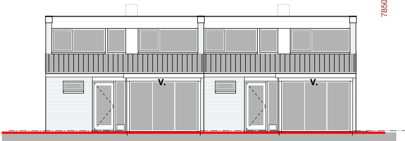
voorgevel
