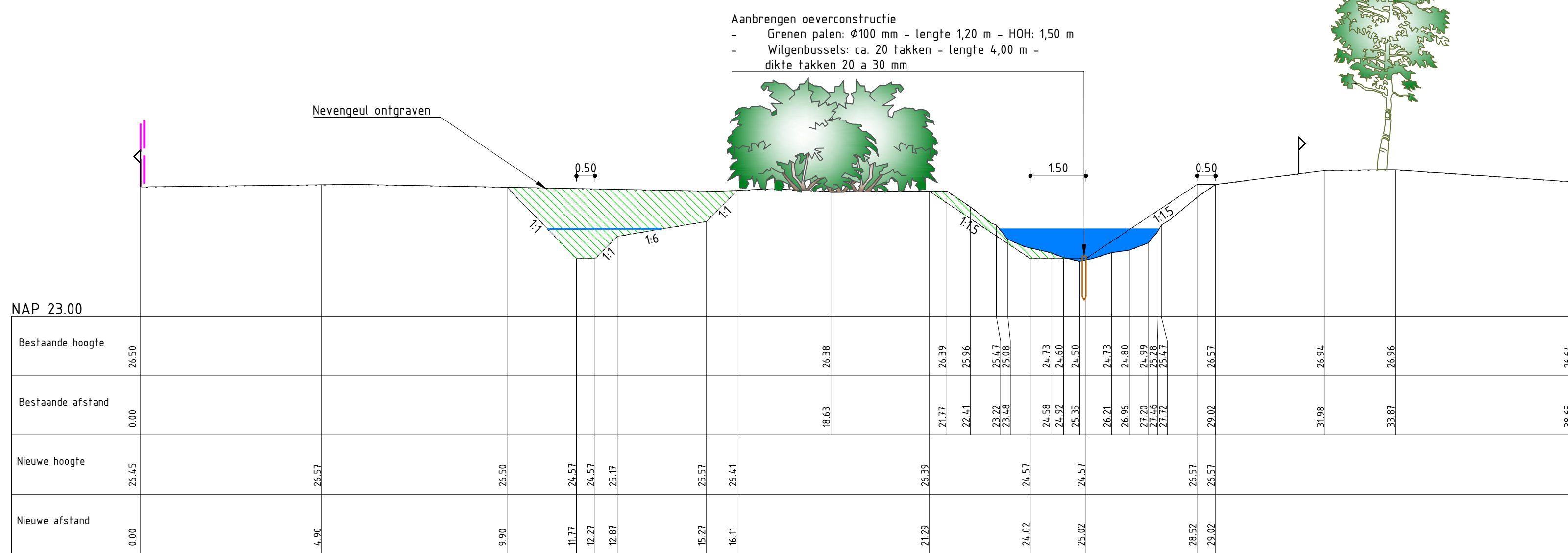
Dwarsprofiel Soeloop So1-So1' (Beekherstel + EVZ)
