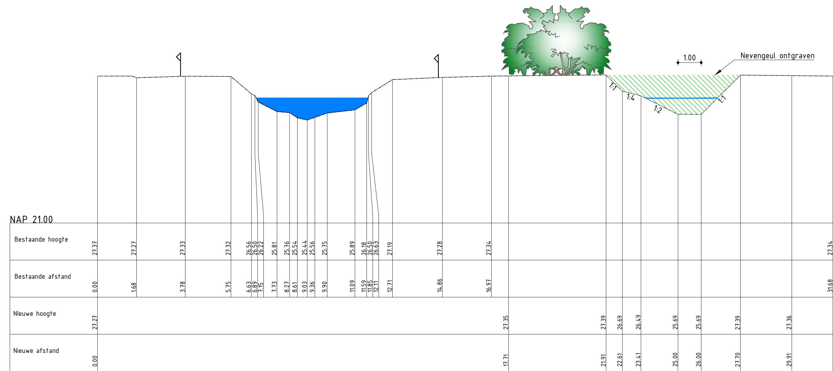
Principeprofiel Soeloop So2-So2' (Beekherstel + EVZ)
