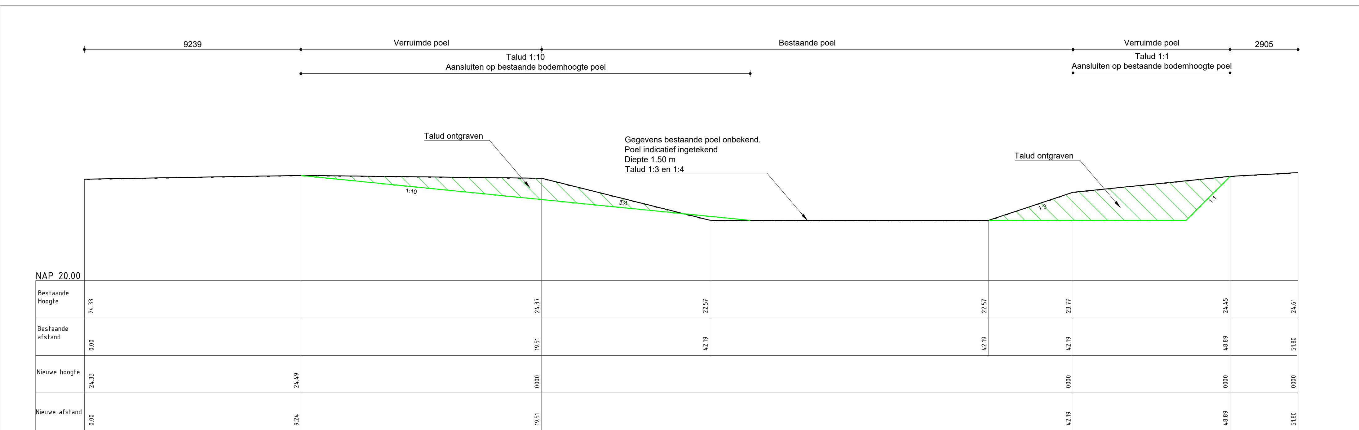
↓Dwarsprofiel Astense AA De Berken Pr1-Pr1' ↑Schaal 1:100
