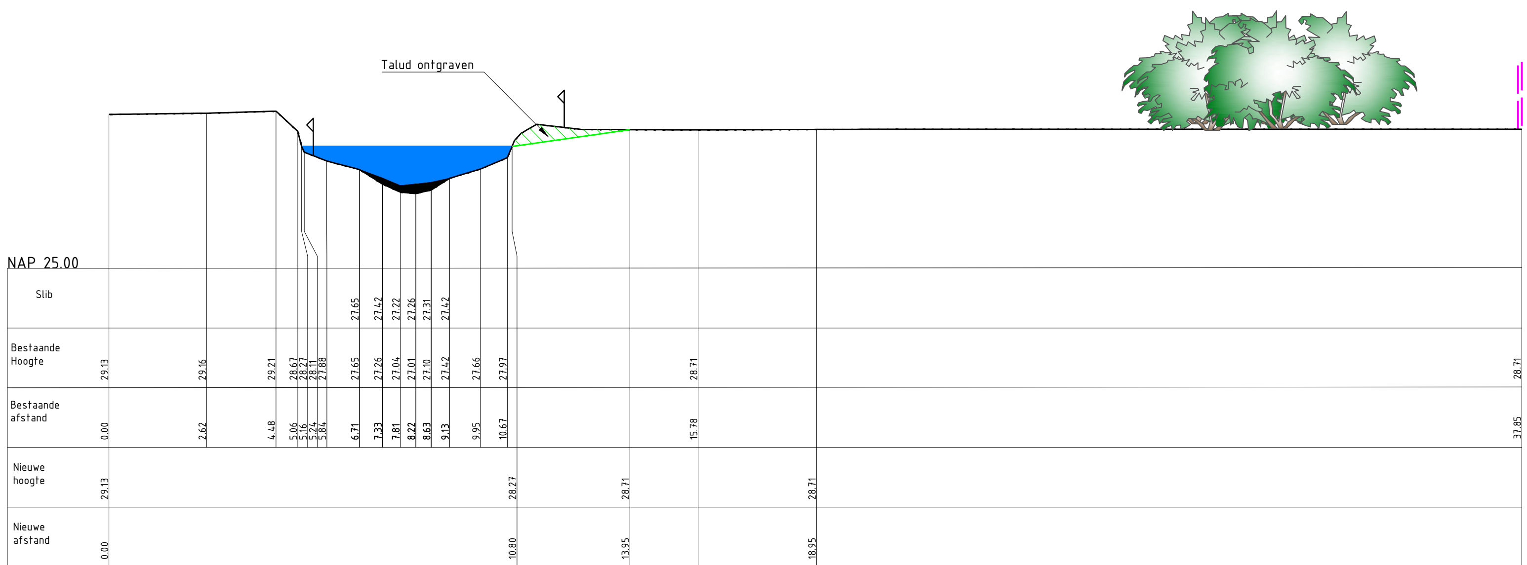
Dwarsprofiel Astense Aa AA6-AA6' (EVZ) Schaal 1:100 Oppervlakte slib: 0,37 m² Dwarsprofiel: 2750010260
