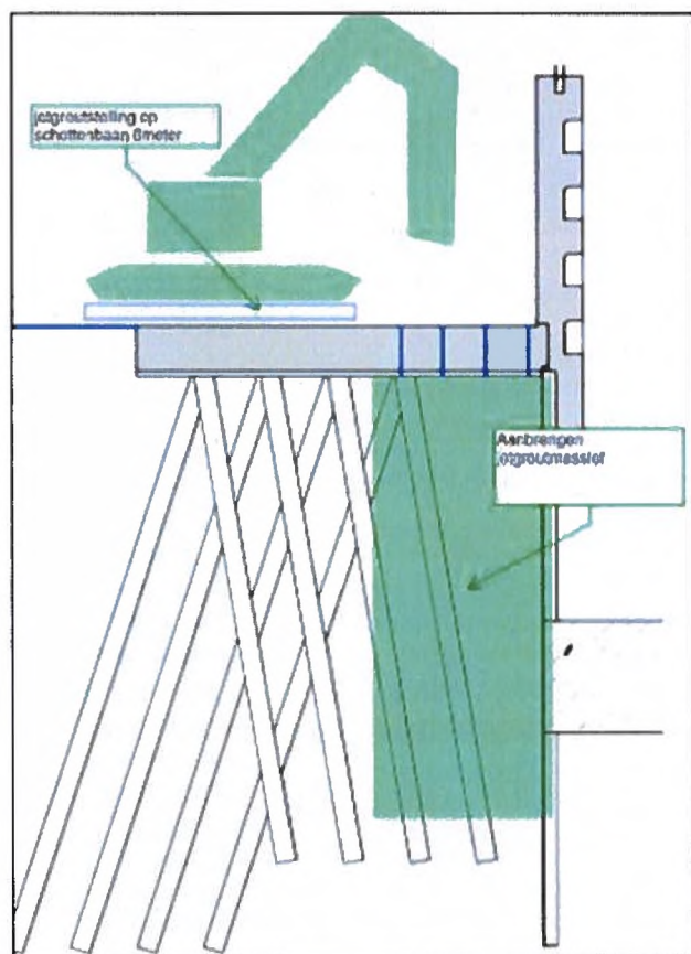
Figuur 2: Schematische weergave van de jetgroutwand (bovenste tekstkader: jetgroutstelling op Schottenbaan 6m, onderste tekstkader: Aanbrengen jetgroutmassief).
