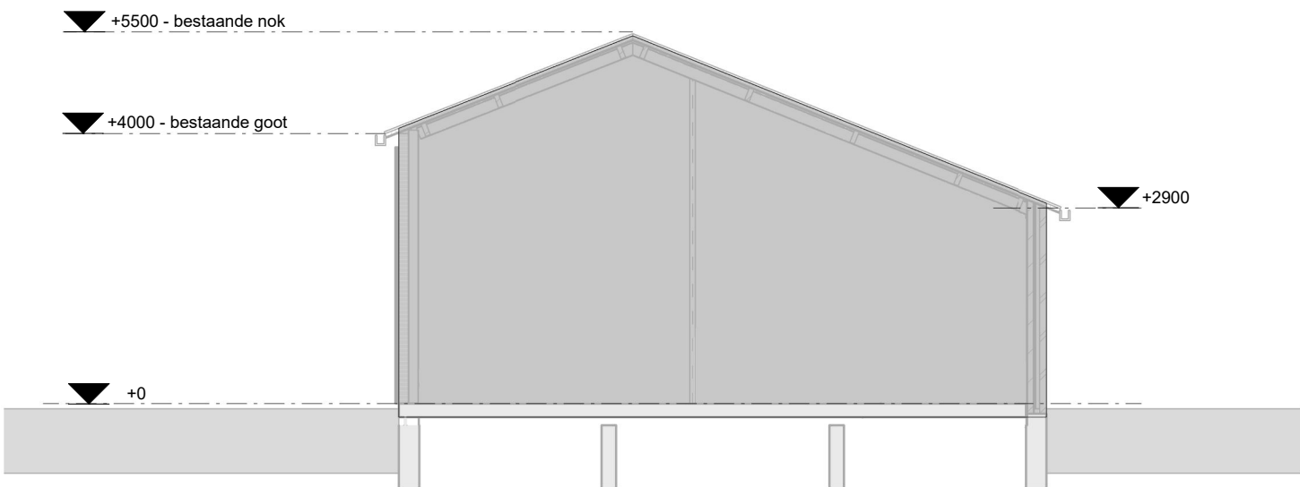
Doorsnede A
