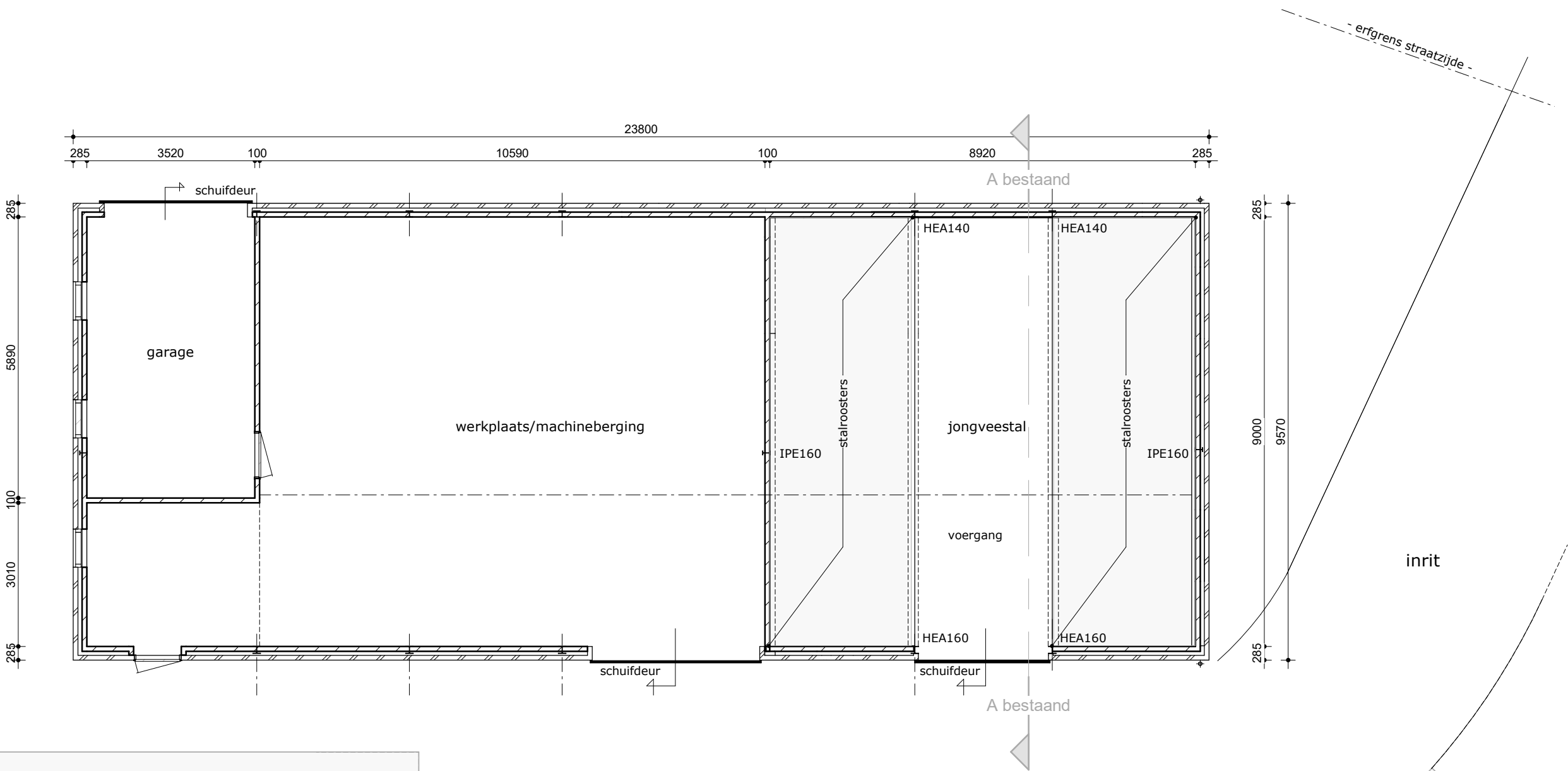
Begane grond - bestaand
