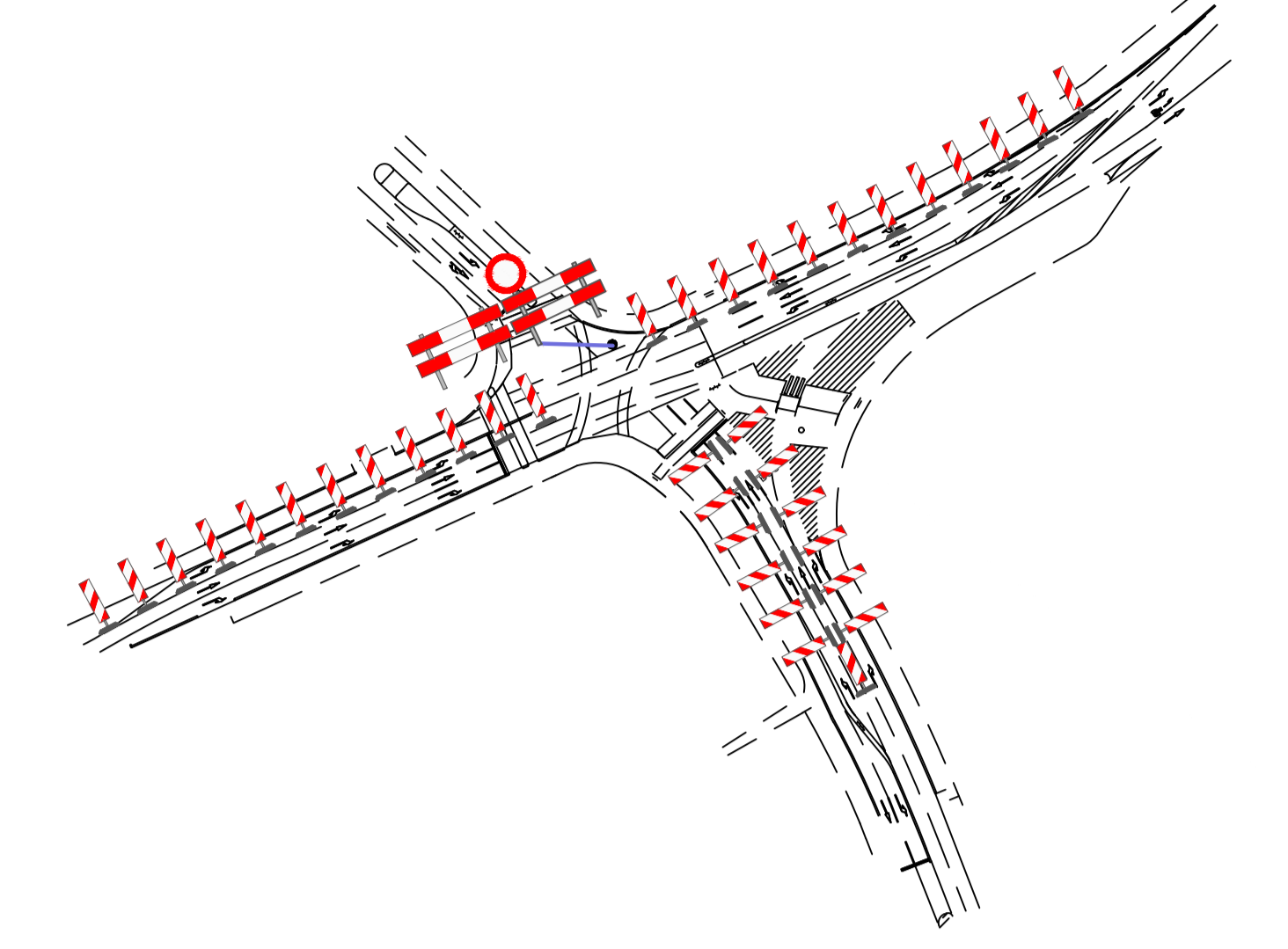
UTSNEDE 1: UITSNEDE MAATREGELEN KRUISSING BODEMPELIN.
