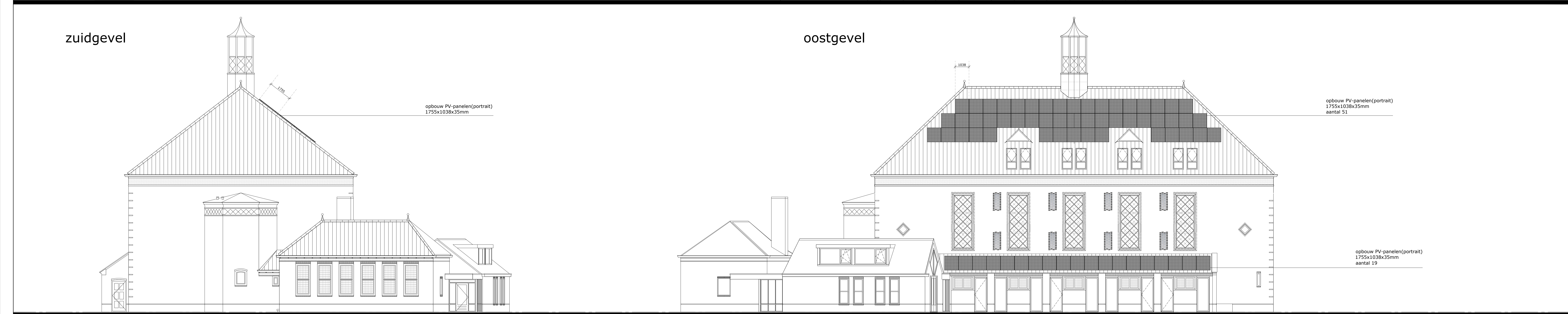
noordgevel
