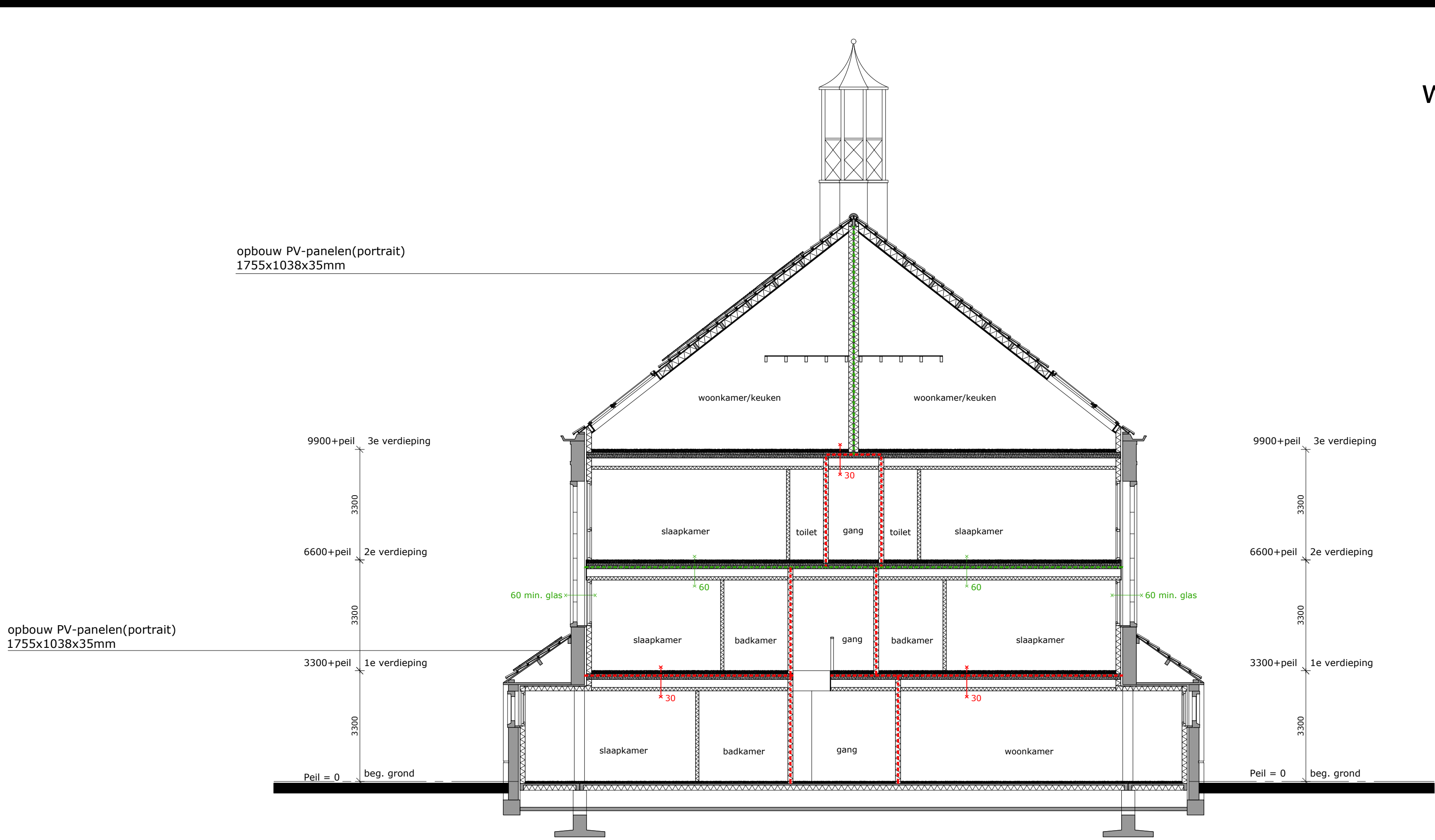
doorsnede A-A
