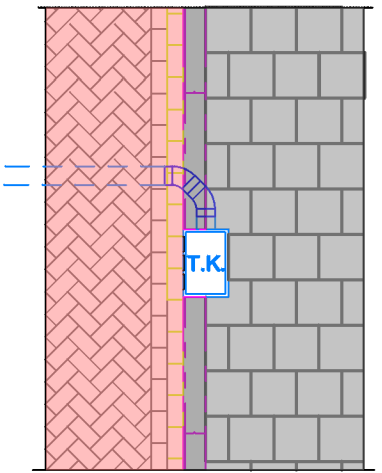
Bovenaanzicht trottoirkolk met kantsteen Kolk met zij-inlaat (alternatief)
