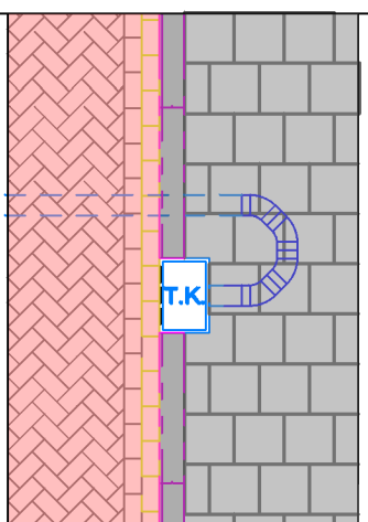
Bovenaanzicht trottoirkolk met kantsteen Kolk met achterinlaat (voorkeur) Kolken aansluiten met bochtstukken van 45 graden
