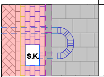
Bovenaanzicht straatkolk in goot achteraansluiting (voorkeur)
