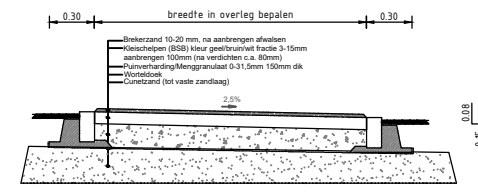
Schikwijdte op uitvoerbaarheid toe laten door Bij gebruik door (onderhouds)voertuigen
