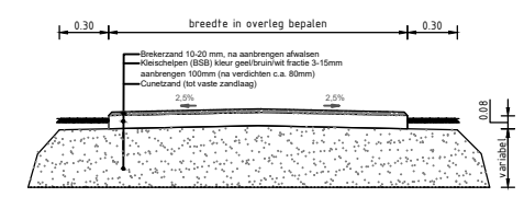
Schikwijdte op constructie (Alleen als het pad gebruikt wordt door voetgangers/fietsers en niet door voertuigen)
