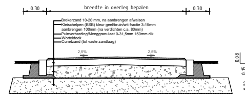
Schikwijdte op uitvoerbaarheid in de praktijk Bij gebruik door (onderhouds)voertuigen
