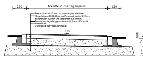
Schikwiel op betonstrook 'n één doer' Bij gebruik door (onderhouds)voertuigen
