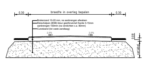
Schikwiel op curietraut (Alleen als het pad gebruikt wordt door voetgangers/fietsers en niet door voertuigen)
