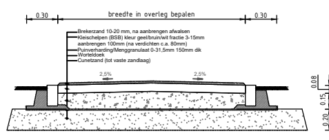
Schikwiel op asfalteerdek Bij gebruik door (onderhouds)voertuigen
