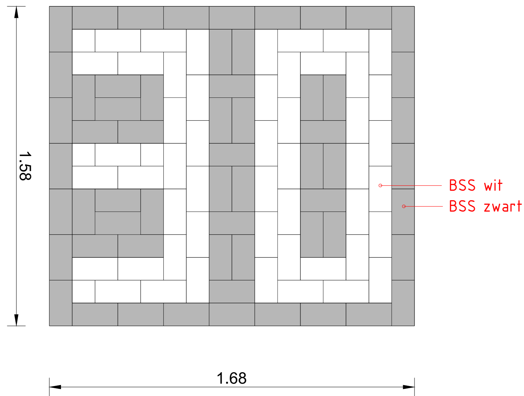
DETAIL 30 km MARKERING Toepassing alleen op verzoek van wegbeheerder.
