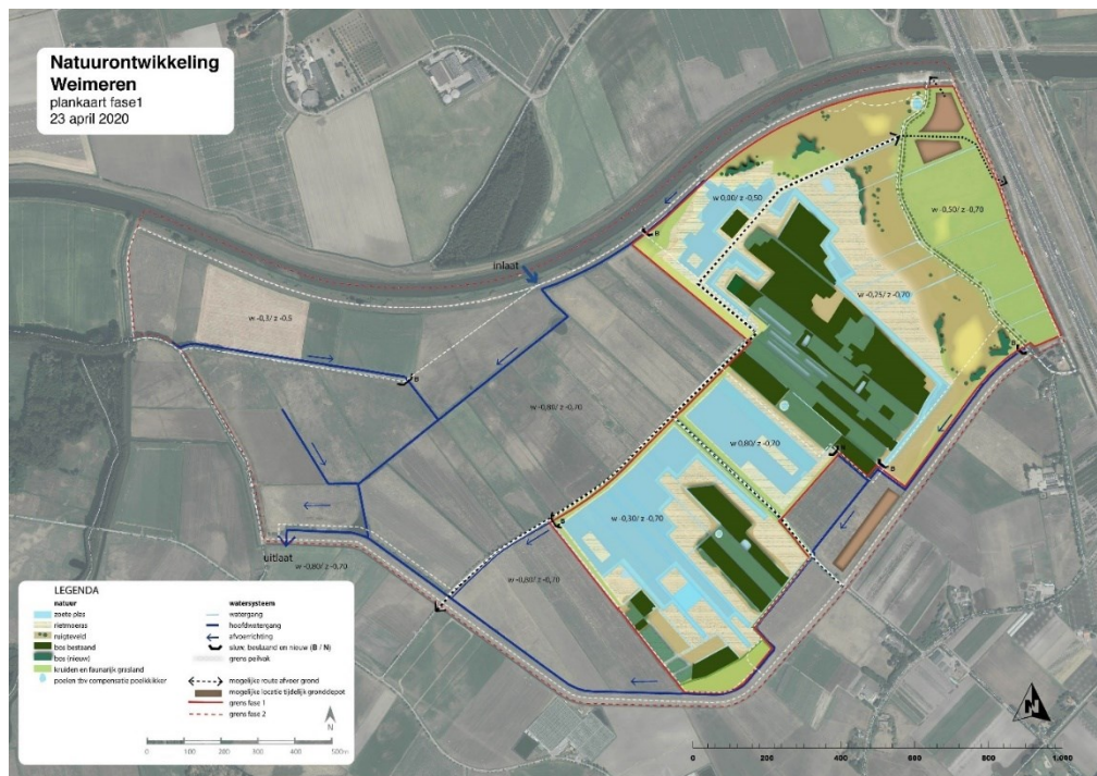
Figuur 1.3: Plangebied en ontwerp Weimeren fase 1
