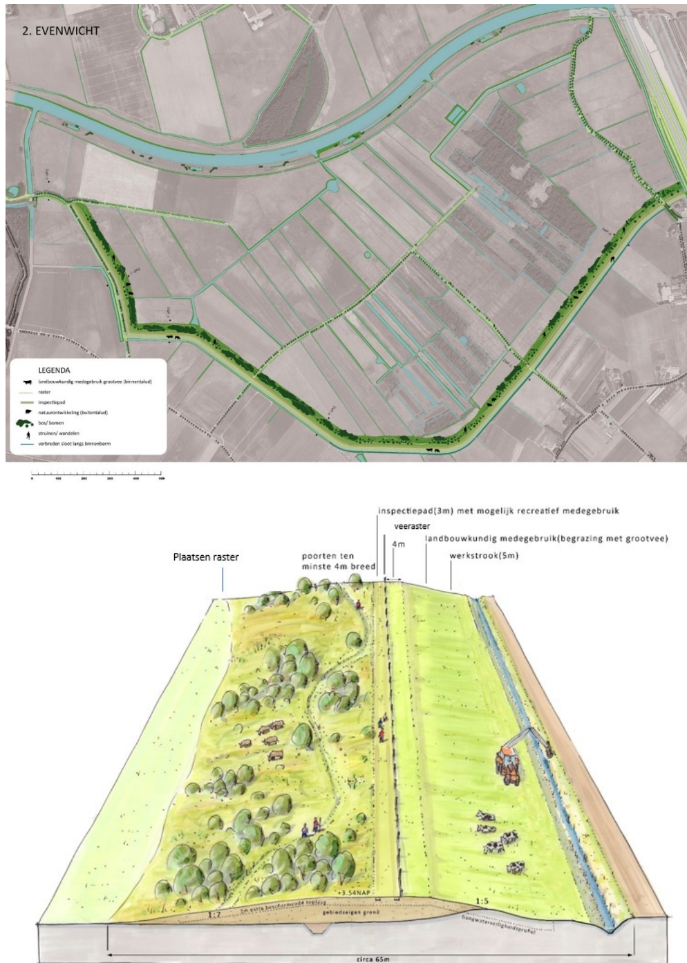
Figuur 1.4: Ruimtebeslag en dwarsdoorsnede verbetering regionale kering Weimeren
