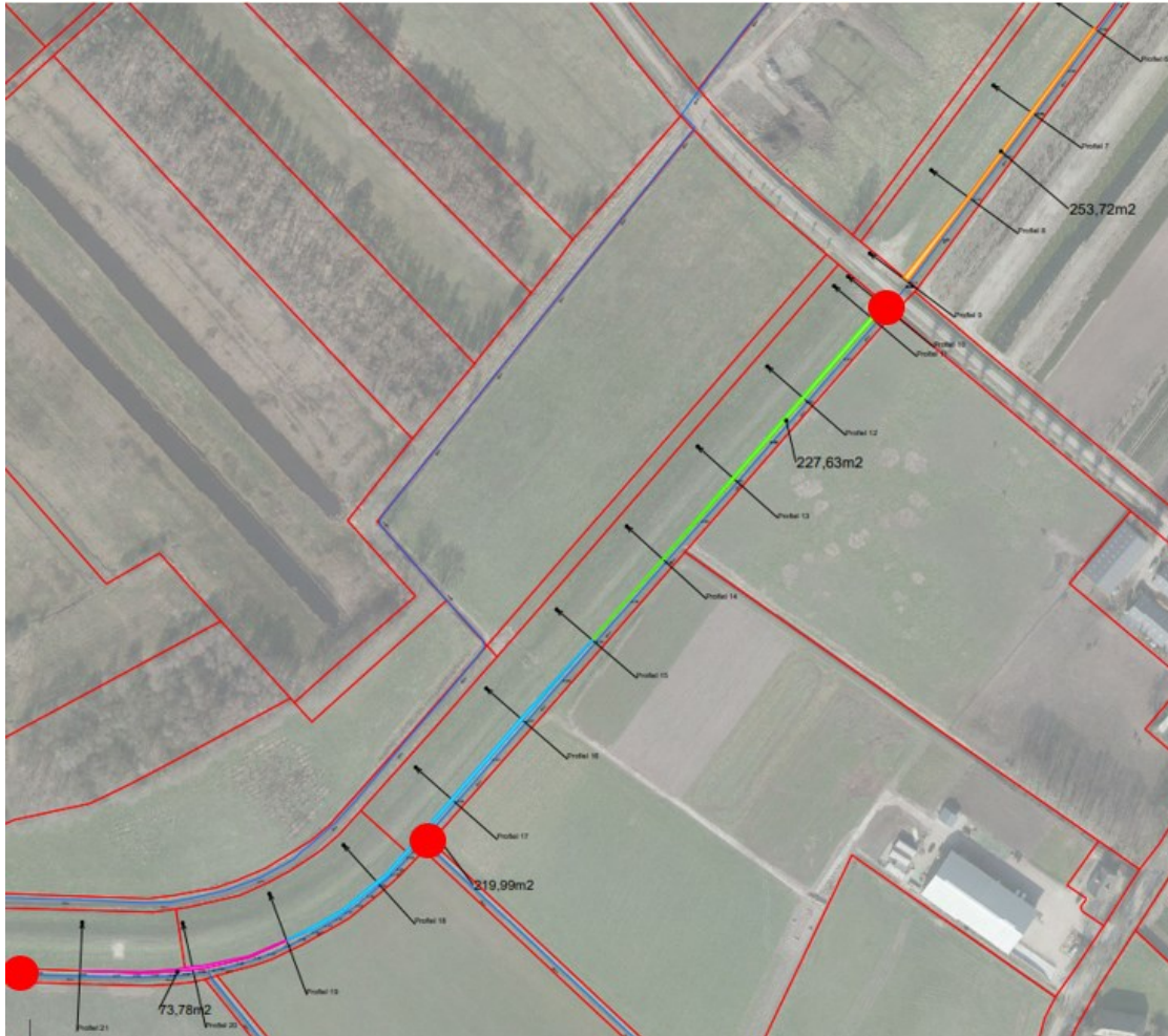
Figuur 4.1.3d: Tracé verbreding teensloot, op de rode stippen worden de duikers aangepast
