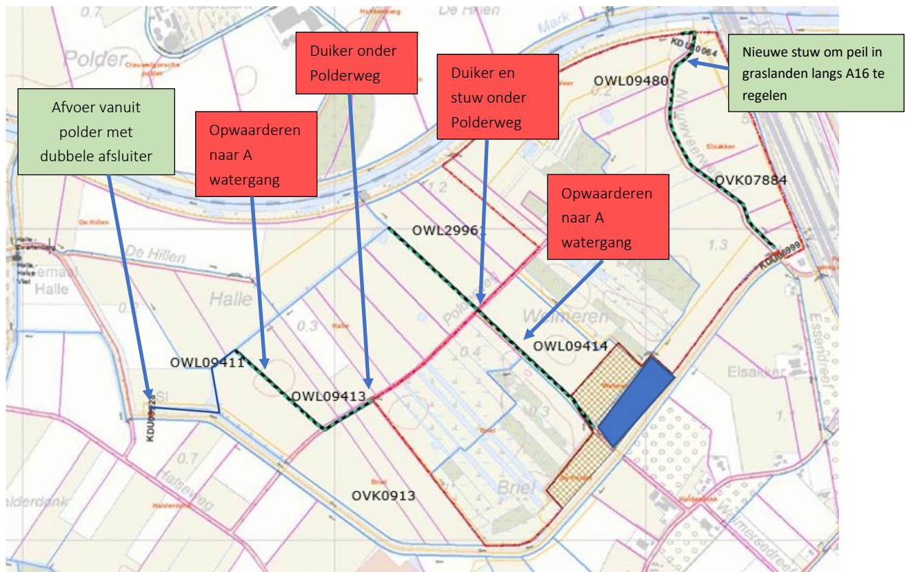
Figuur 4.3b: Uit projectplan waterwet Kering Weimeren . Overzicht aanpassingen tijdelijke waterhuishouding Weimeren t.b.v. landbouw Weimeren fase 1. De tijdelijke situatie vervalt bij inrichting percelen fase 2. In het groen de maatregelen die behouden blijven in dit projectplan, in het rood de maatregelen die komen te vervallen.
