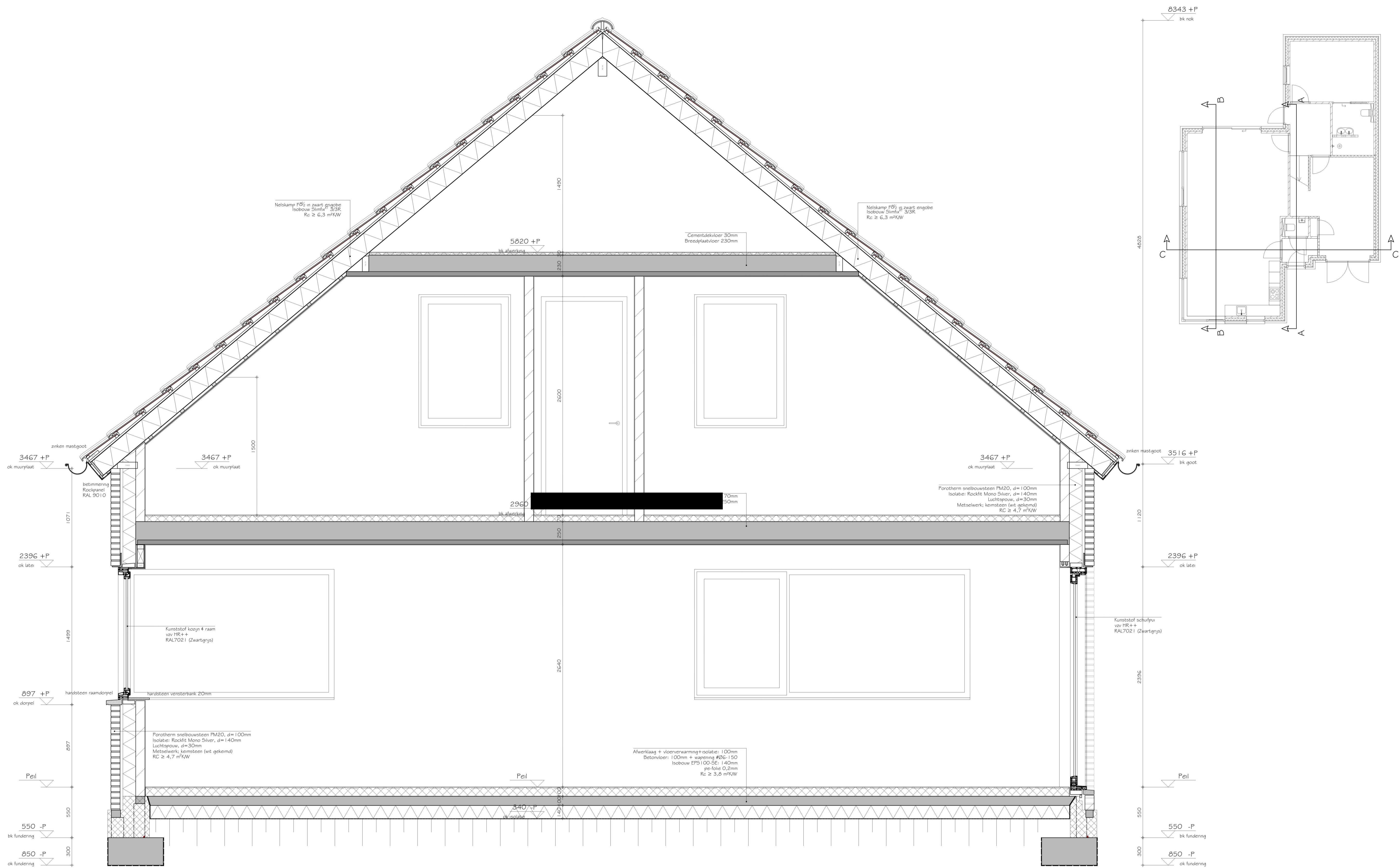
DOORSNEDE B-B
