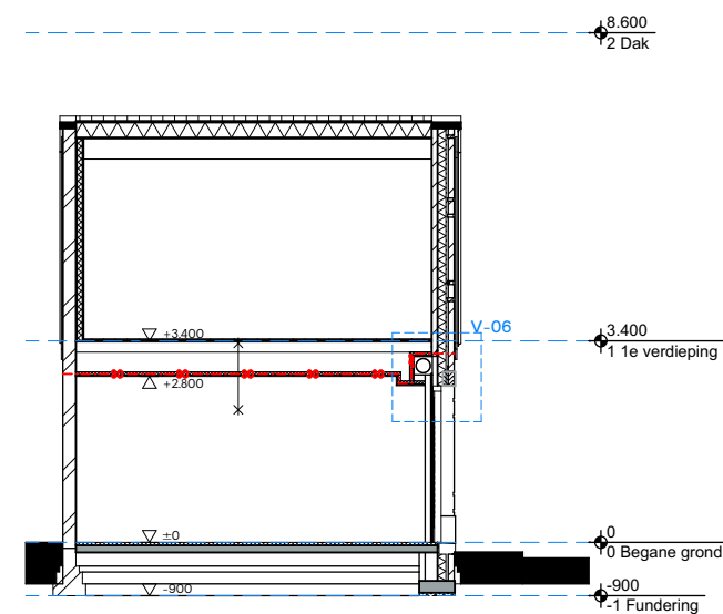
Doorsnede C
