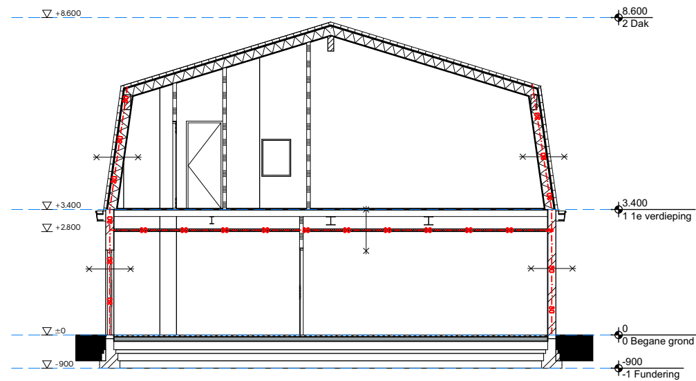
Doorsnede F
