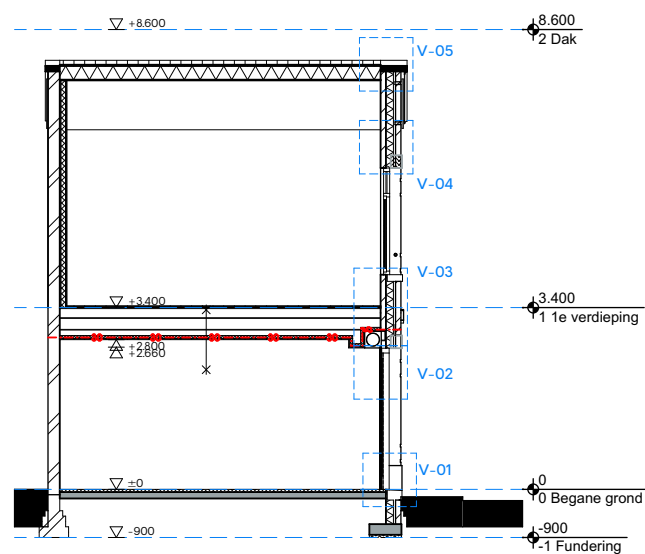
Doorsnede B
