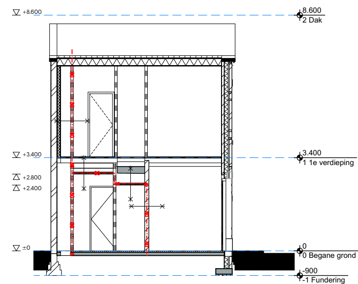
Doorsnede A
