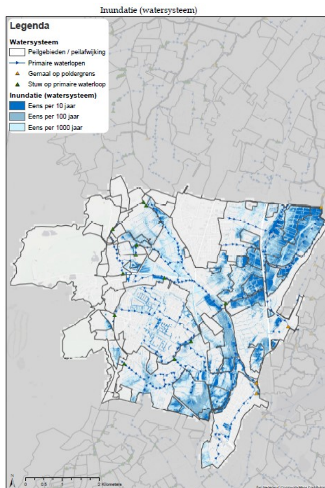
Figuur 5: Inundatie vanuit het watersysteem
