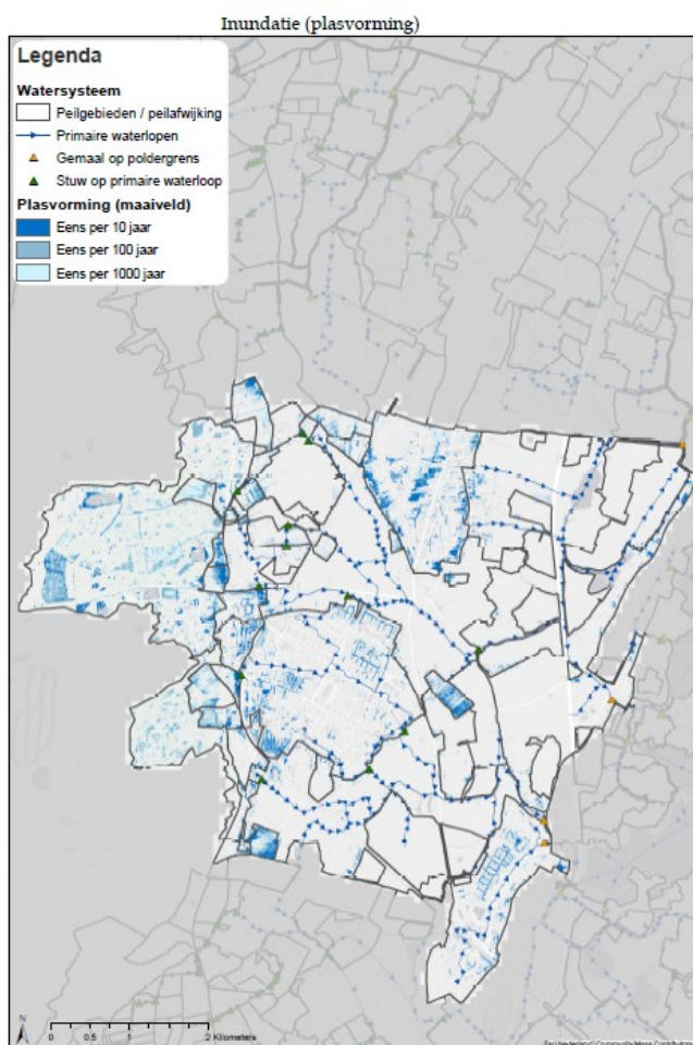
Figuur 4: Inundatie als gevolg van plasmvorming
