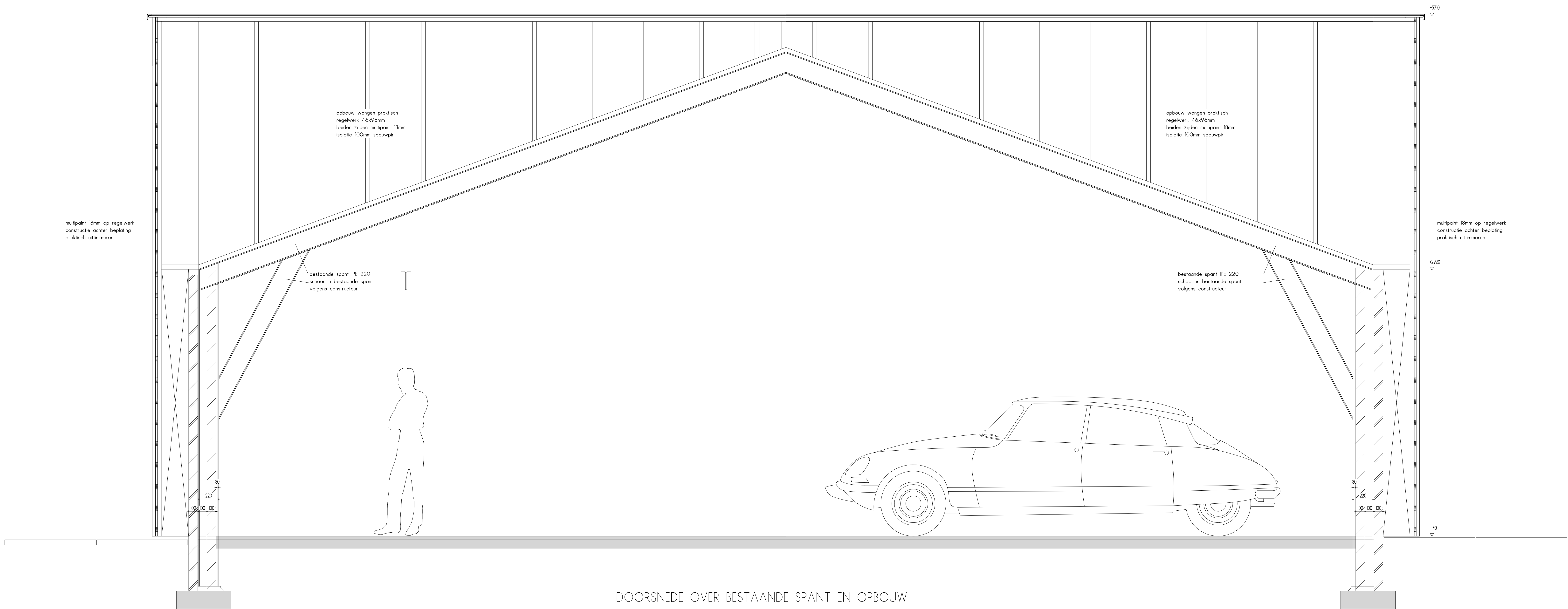
DOORSNEDE OVER BESTAANDE SPANT EN OPBOUW
