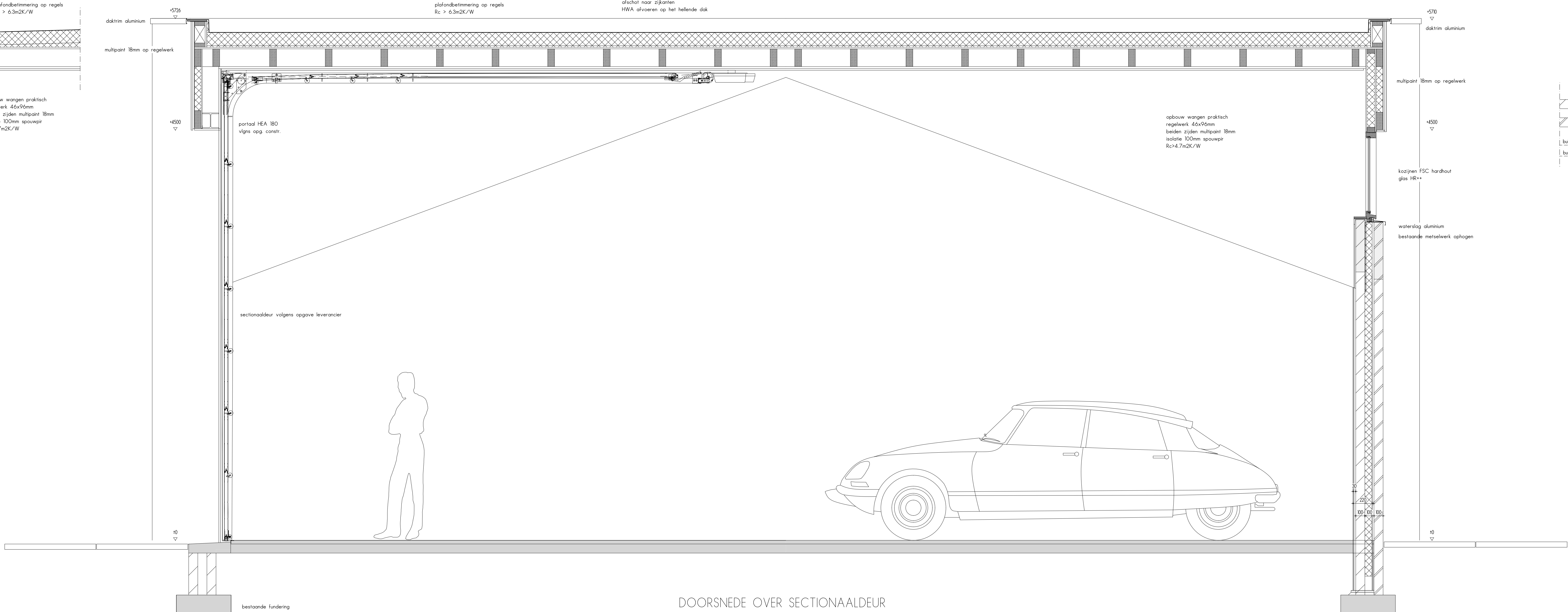
DOORSNEDE OVER SECTIONAALDEUR
