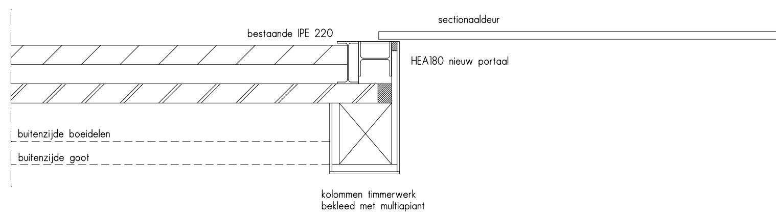
DETAILS HORIZONTAAL
