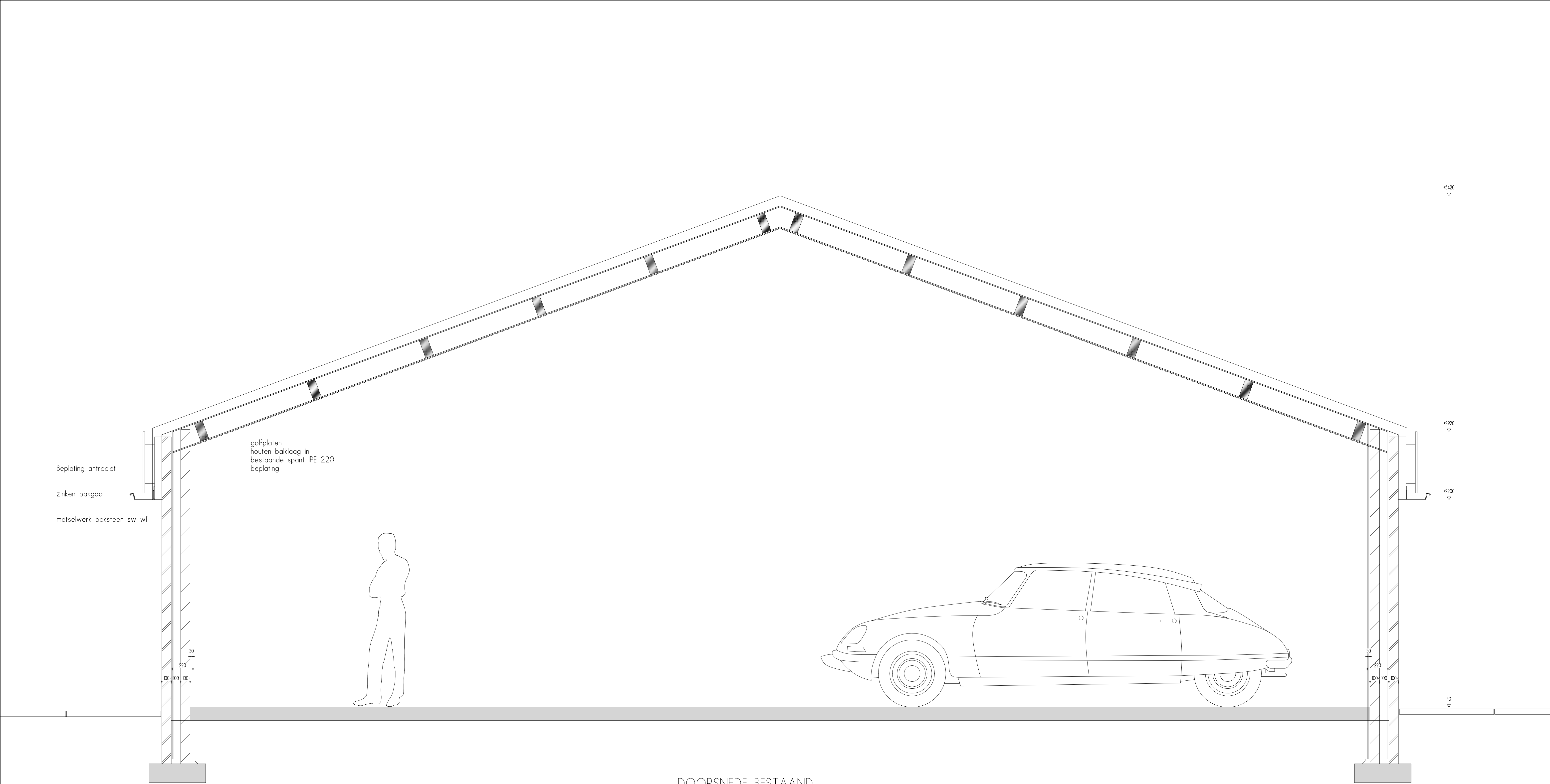
DOORSNEDE BESTAAND
