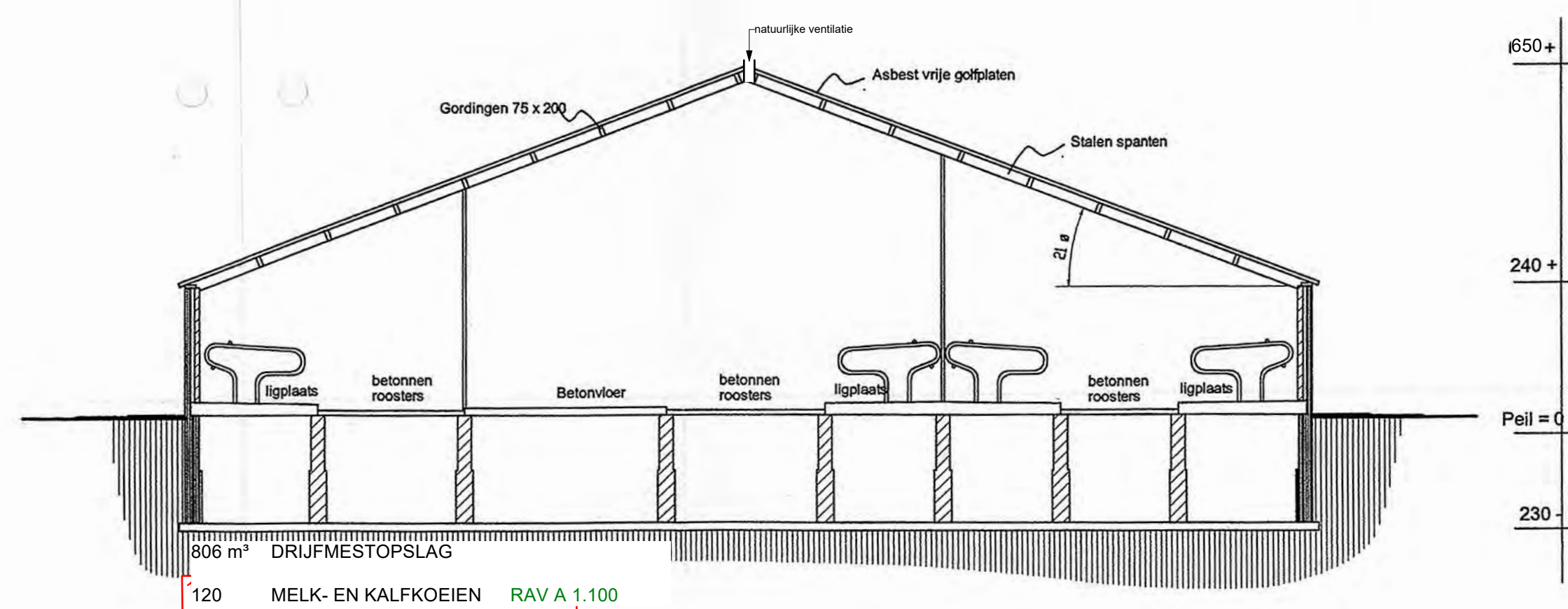
Doorsnede C-C Stal D
