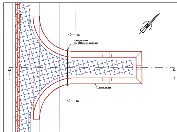
SITUATIE KEERLUS MOF 5 SCHAAL 1:200
