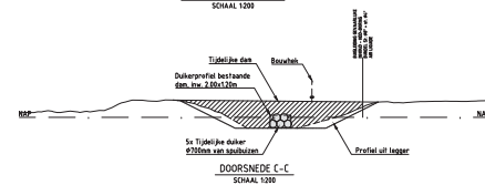
DOORSNEDE C-C SCHAAL 1:200
