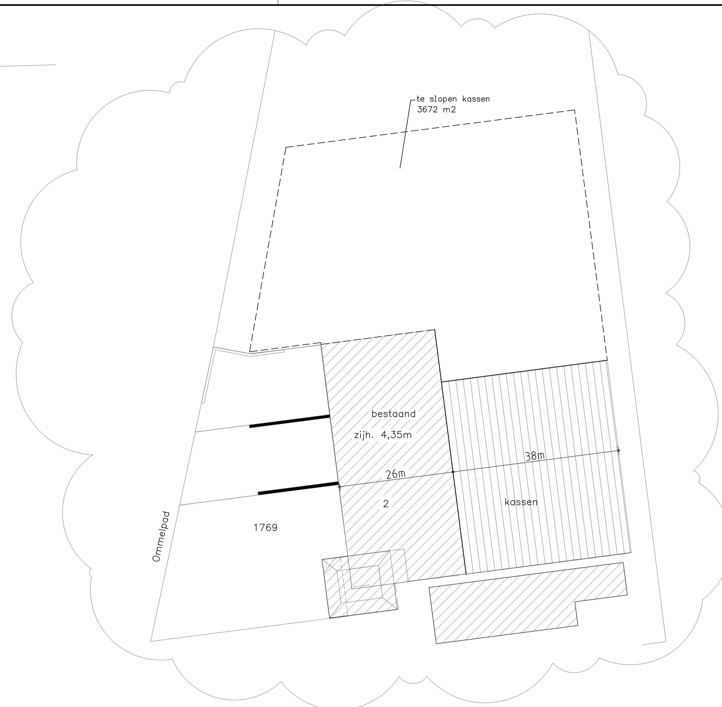
SITUATIE Bestand
