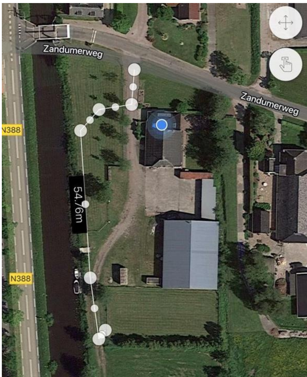
Figuur 1: De witte bolletjeslijn geeft de ligging van de nieuwe oprit weer. De kern- en beschermingszone van de waterkering reikt tot ongeveer 11 meter uit de oever van het Wolddiep.
