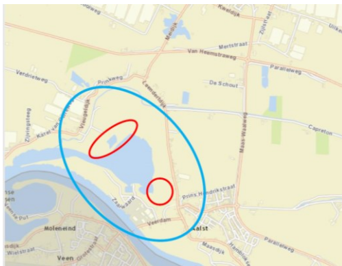
Figuur 1 Globale ligging van de 2 deelgebieden
